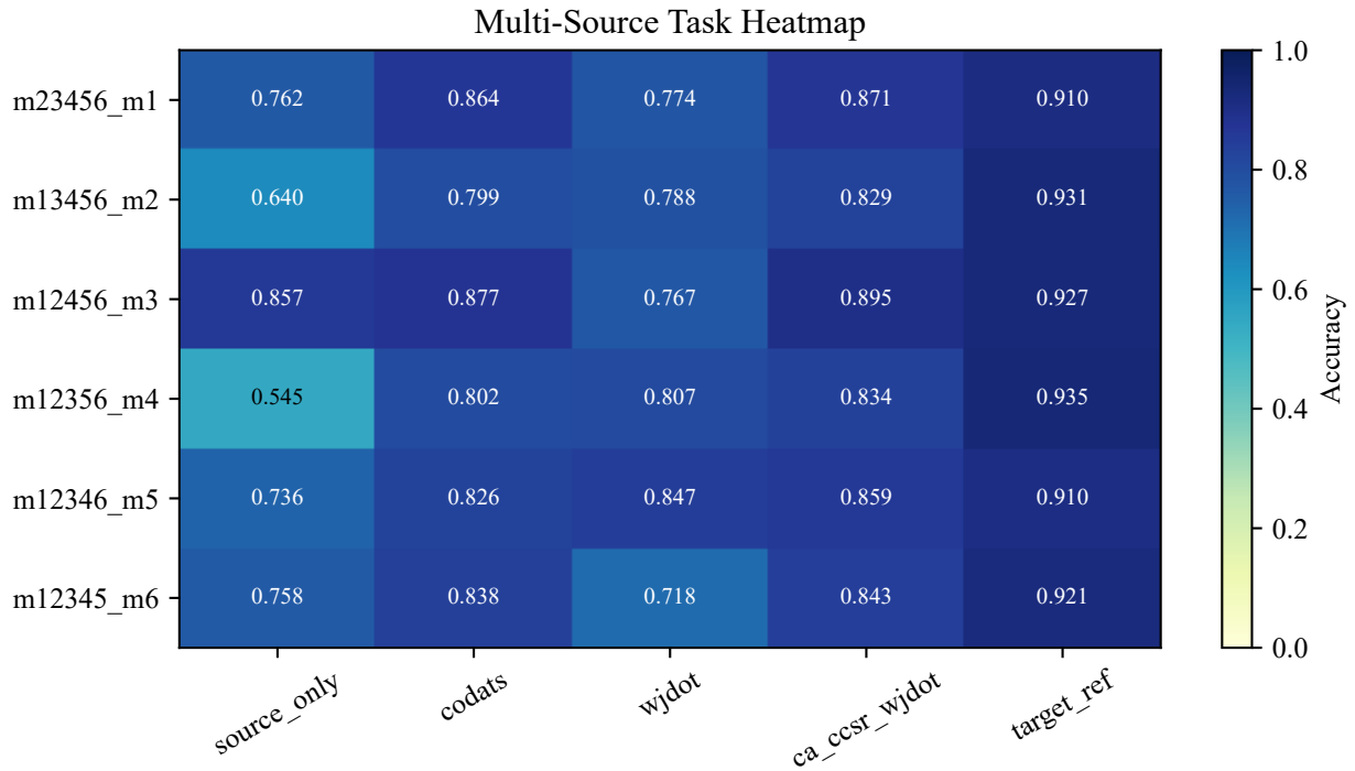
图 6-5 五源留一域逐目标生产模式准确率热力图
