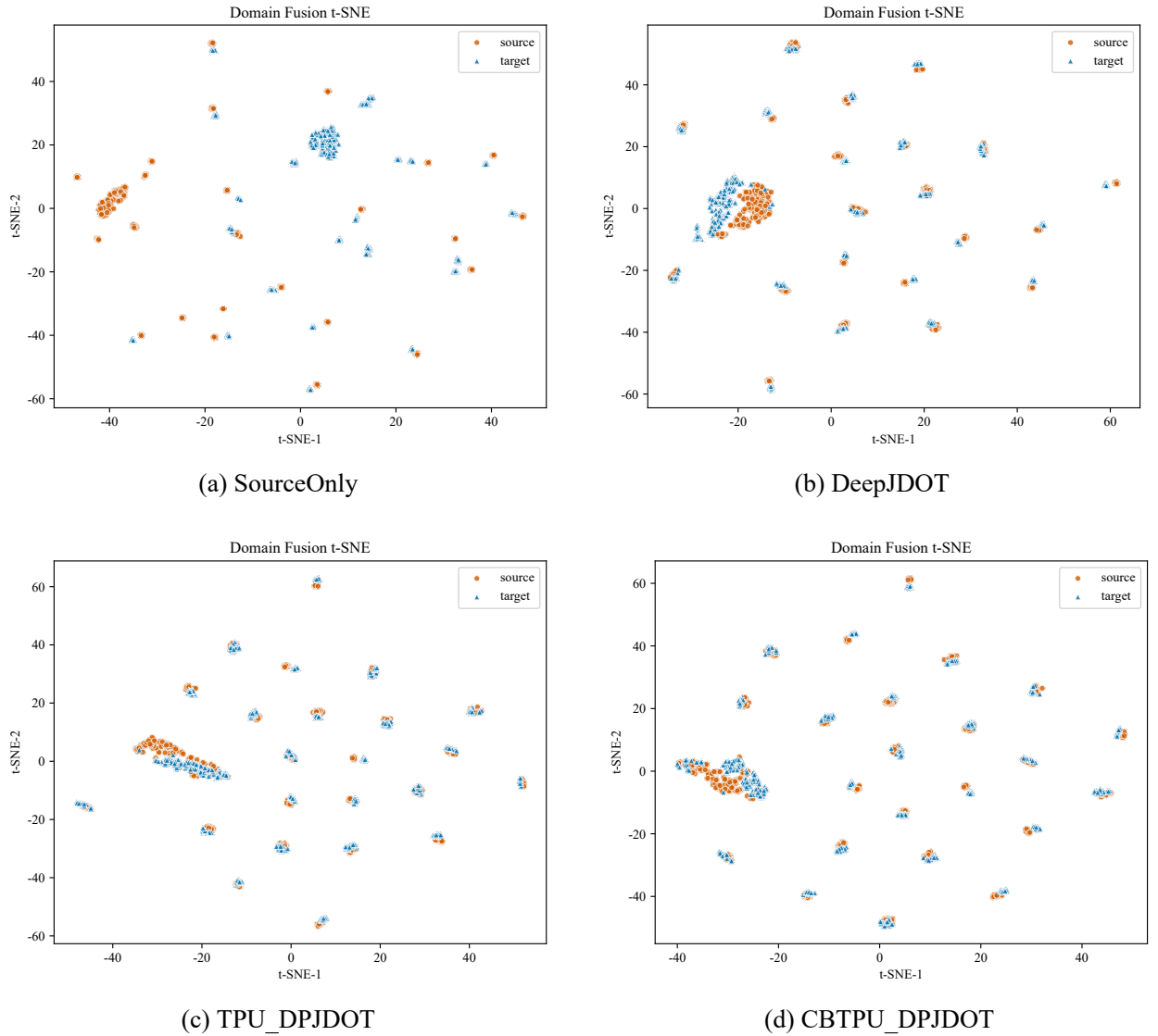
图 6-4 单源任务 m_5 \rightarrow m_2 中单源主线方法的域融合特征可视化
