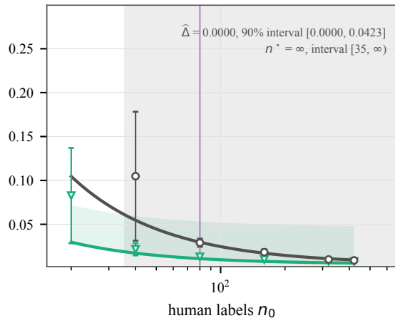
PandaLM (pilot n_0 = 80 )
