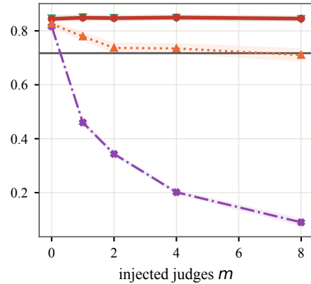
(d) position-only, Kendall \tau
