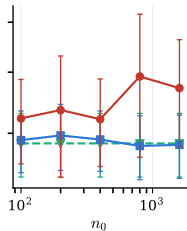
RMSE( \hat{b}, b )
