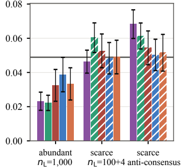
(g) PandaLM, n_H=60
