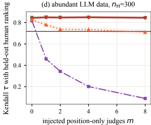
(d) abundant LLM data, n_H=300
