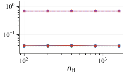
RMSE( \hat{b}, b )
