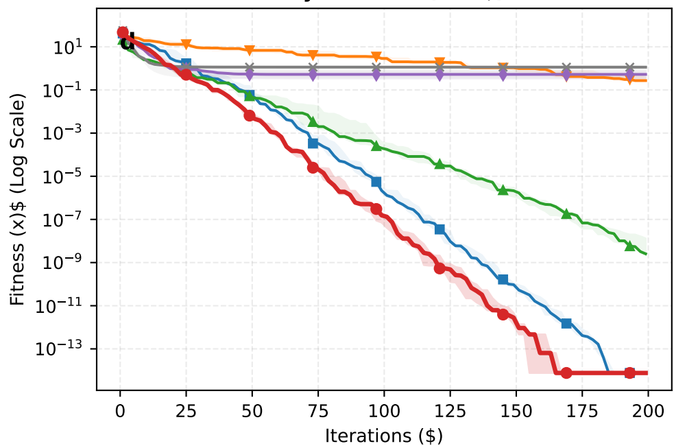
Levy Function (=10$)
