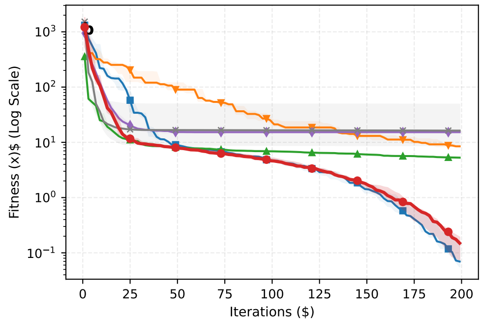
Levy Function (=10$)
