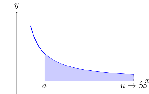
图 2.1: 无穷区间积分的示意图
