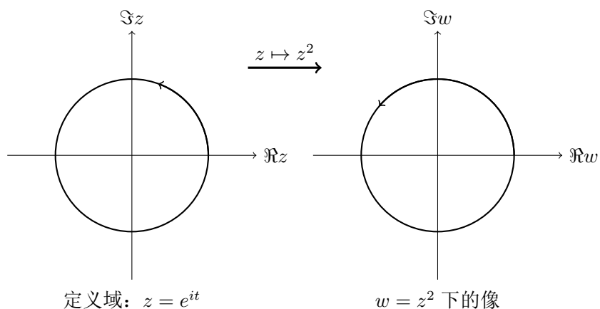
图 7.1: 映射 z \mapsto z^2 使辐角加倍. z 平面中一段圆弧的一次运动, 会在 w 平面中产生两倍的角度变化。
