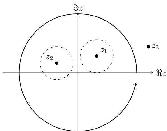
图 7.2: 留数围道包含 z_1 与 z_2 , 但不包含 z_3 . 围道积分等于所包围奇点留数之和的 2\pi i 倍, 其中还要计入绕数。
