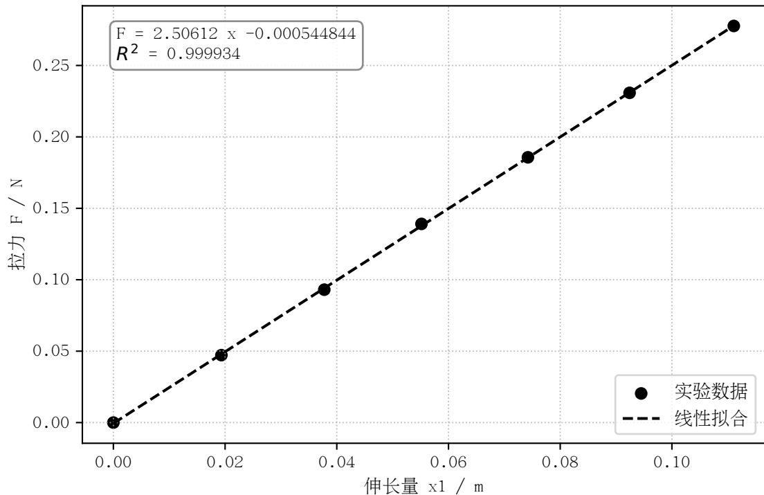
实验1：弹簧1 静态拉伸拟合
