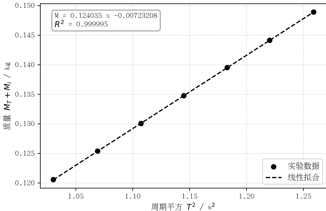
实验2：周期平方与质量关系拟合
