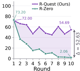
(d) Majority Accuracy (%)
