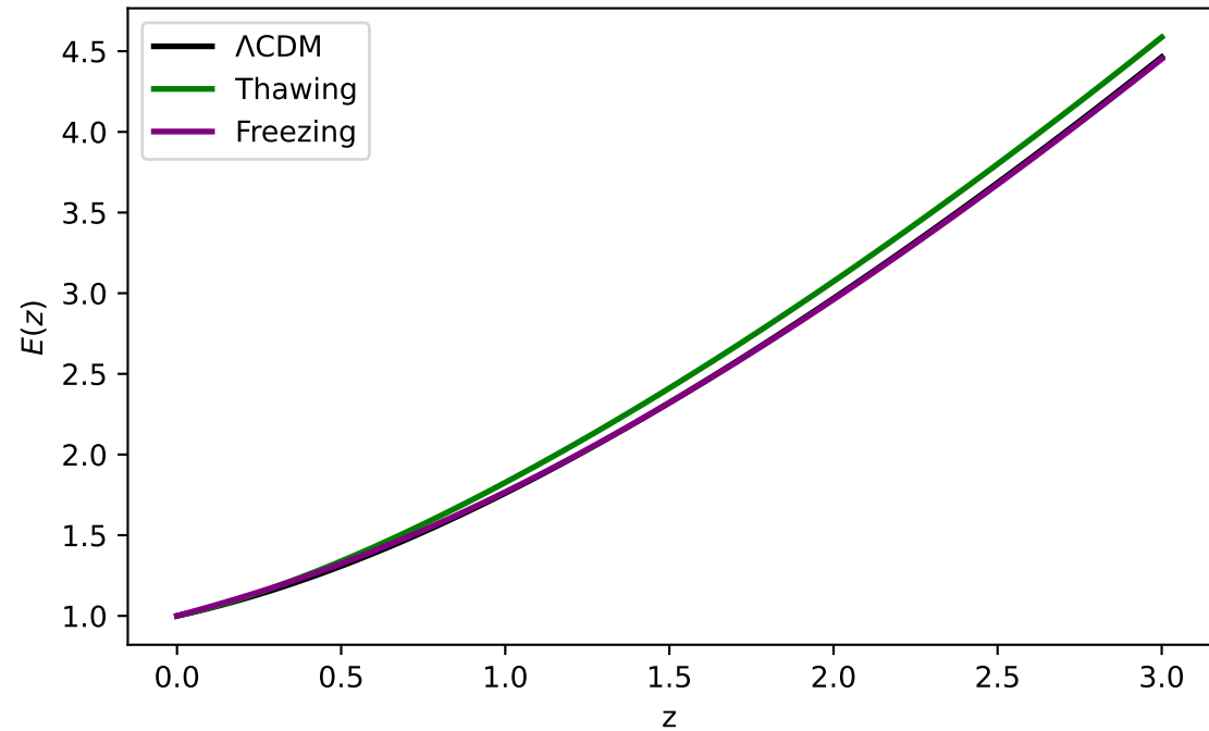
Hubble Parameter
