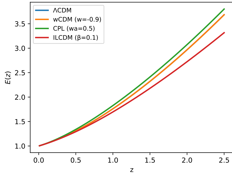
Hubble Parameter
