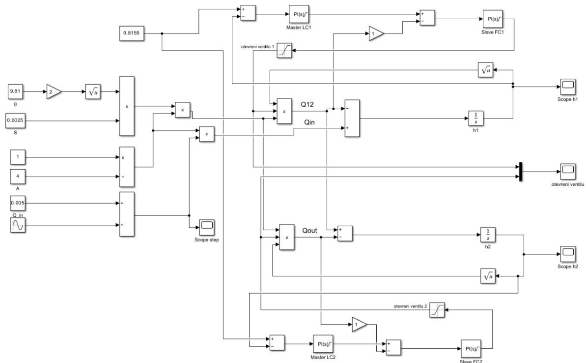
Obr. 12 – SIMULINK model k úkolu 4
