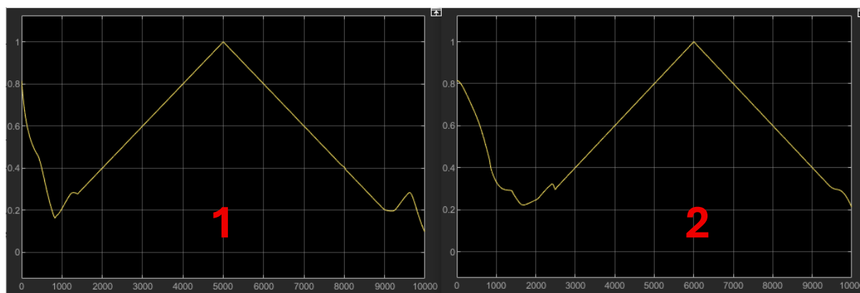
Obr. 22 – Průběh regulace hladin nádrží 1 (graf 1) a 2 (graf 2) pomocí master-slave regulace
