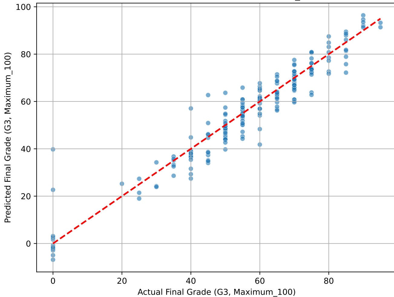
Actual G3 vs. Predicted G3 (Maximum_100)
