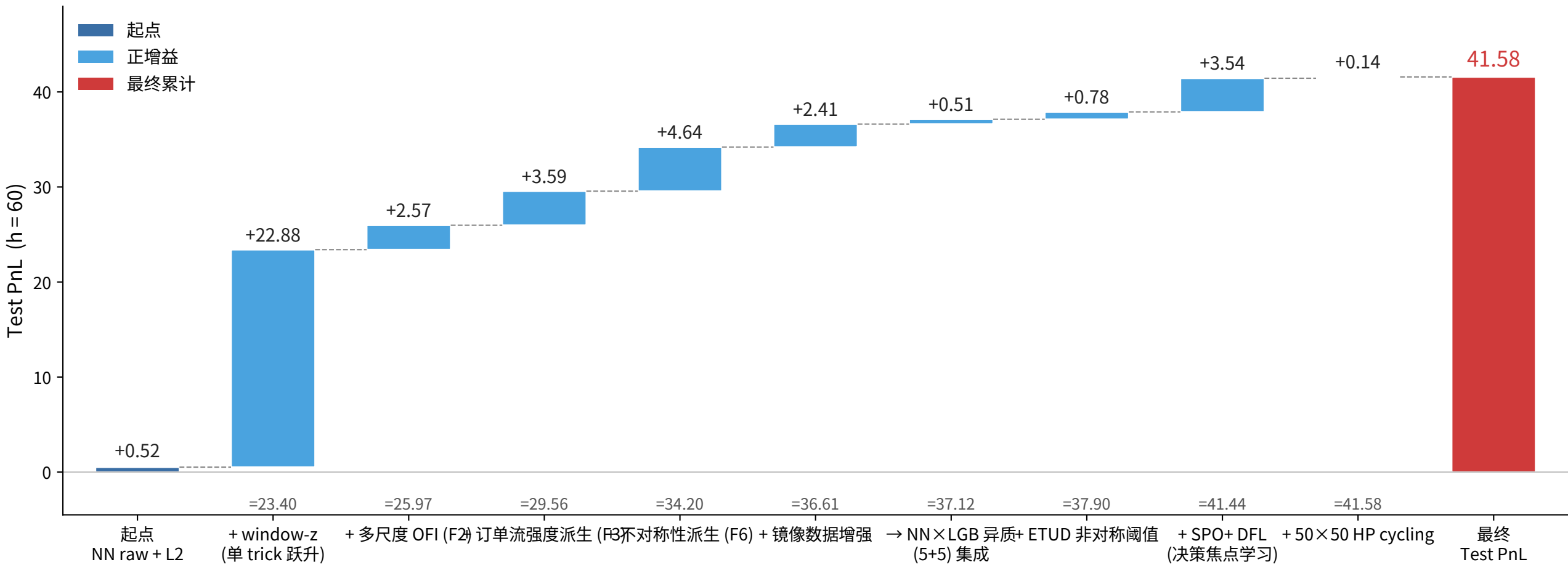
关键 trick 增益 waterfall —— 起点 NN raw+L2 (0.52) → 集成最终 41.58
