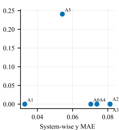
Gibbs-Duhem
