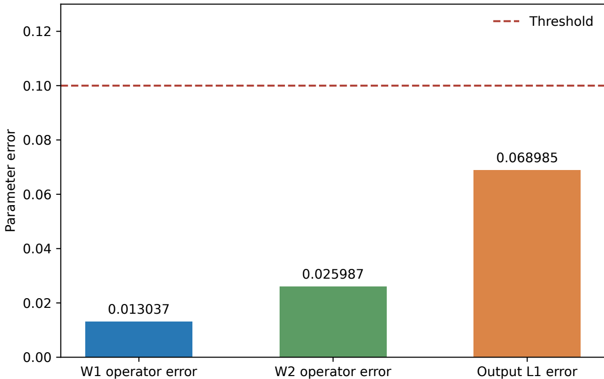
Experiment (k=4): aligned parameter errors
