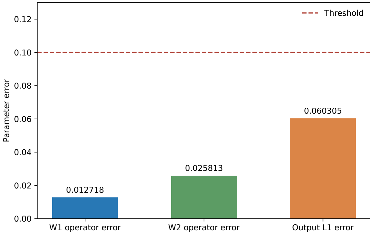
Experiment (k=6): aligned parameter errors
