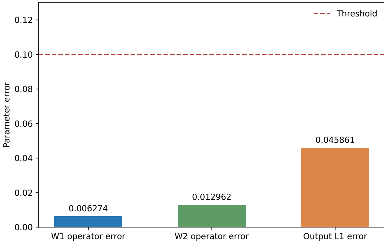
Experiment 1 (k=8): aligned parameter errors
