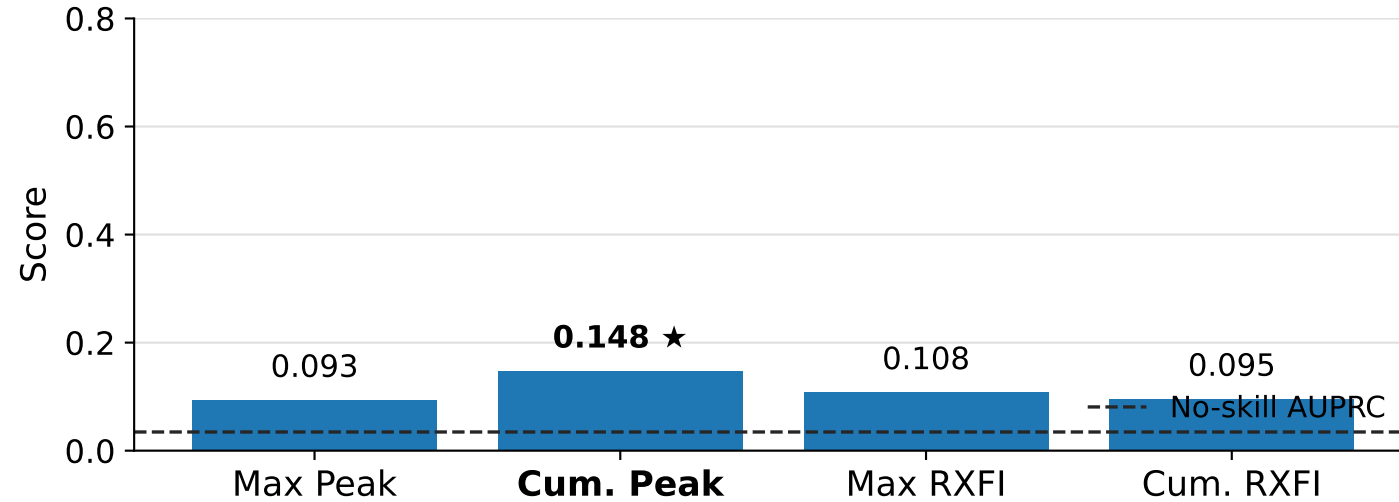
AUPRC
