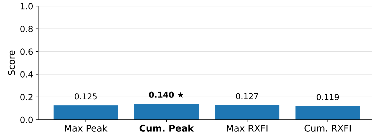
Positive F1
