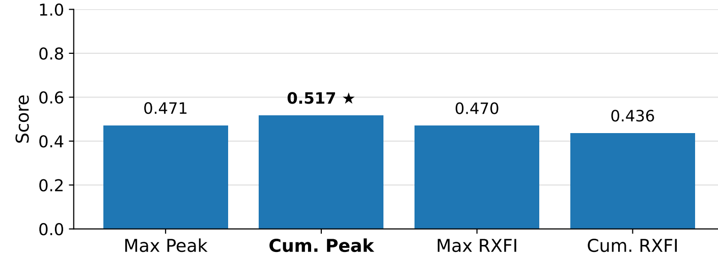
TSS
