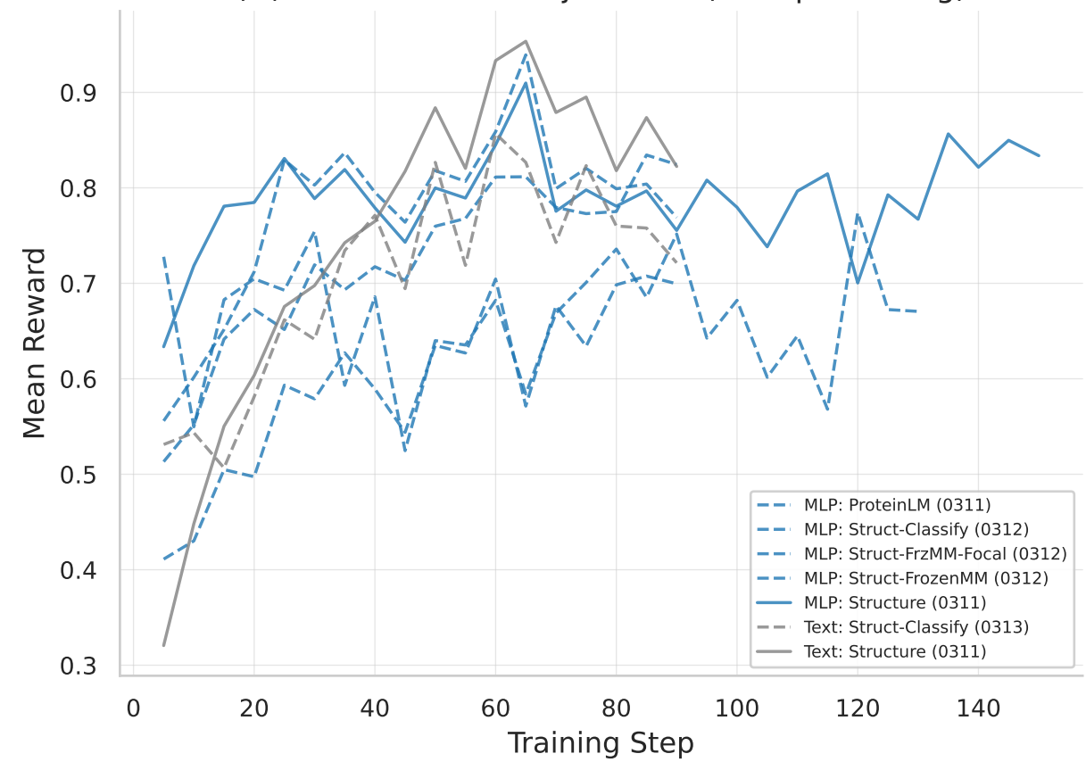
(D) GRPO Reward Trajectories (Best per Config)
