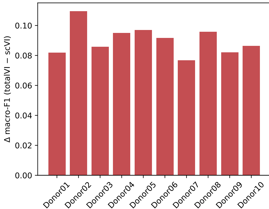
Donor-level \Delta F1
