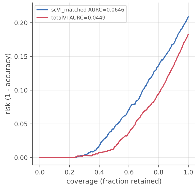
A: PBMC10k \rightarrow PBMC5k
