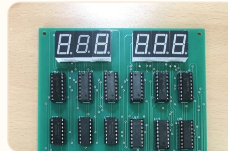
조립 · 납땀한 회로 기판
