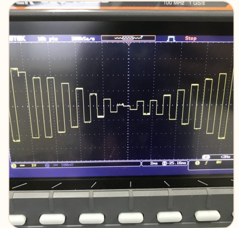
파형 측정 (고장수리)
