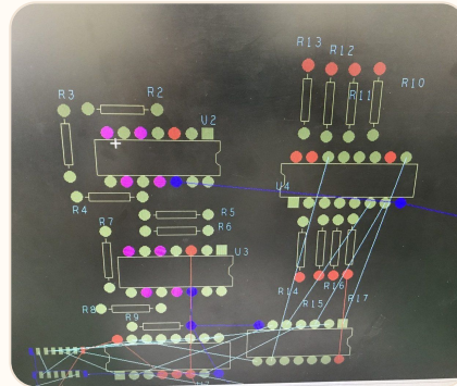
PCB CAD 배치 작업
