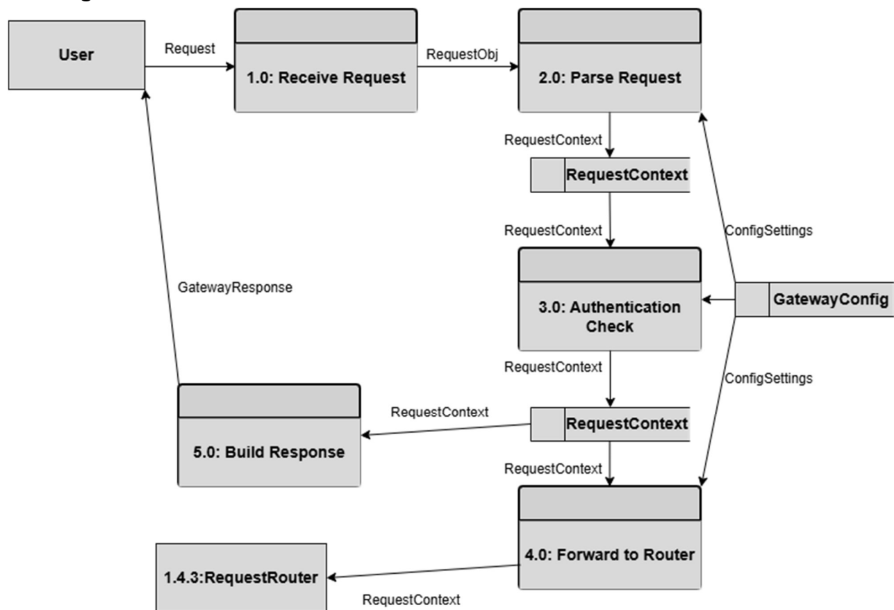
DFD Figure – 1.4.1.0.1 –
