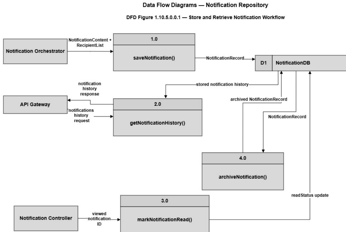
DFD Figure 1.10.5.0.0.1
