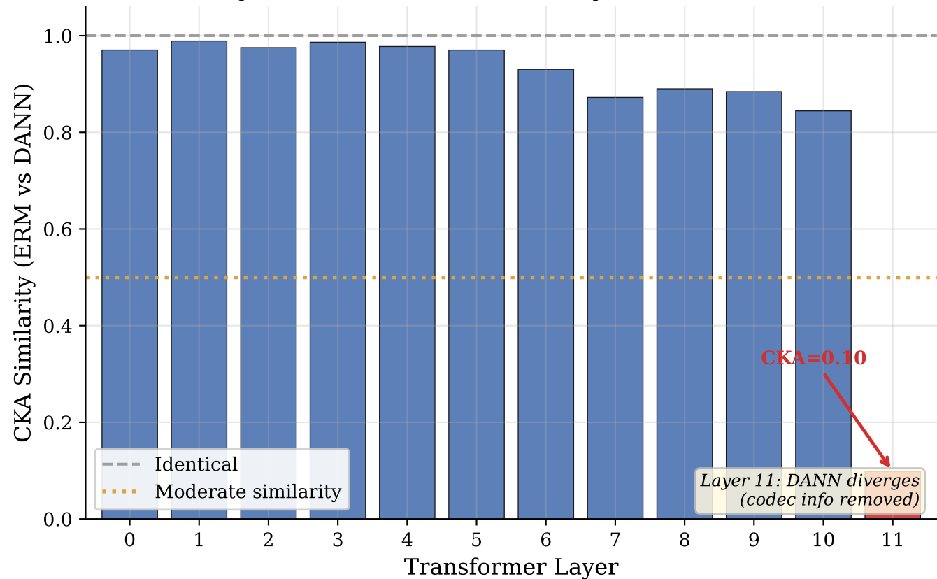
Layer Contribution Similarity: ERM vs DANN
