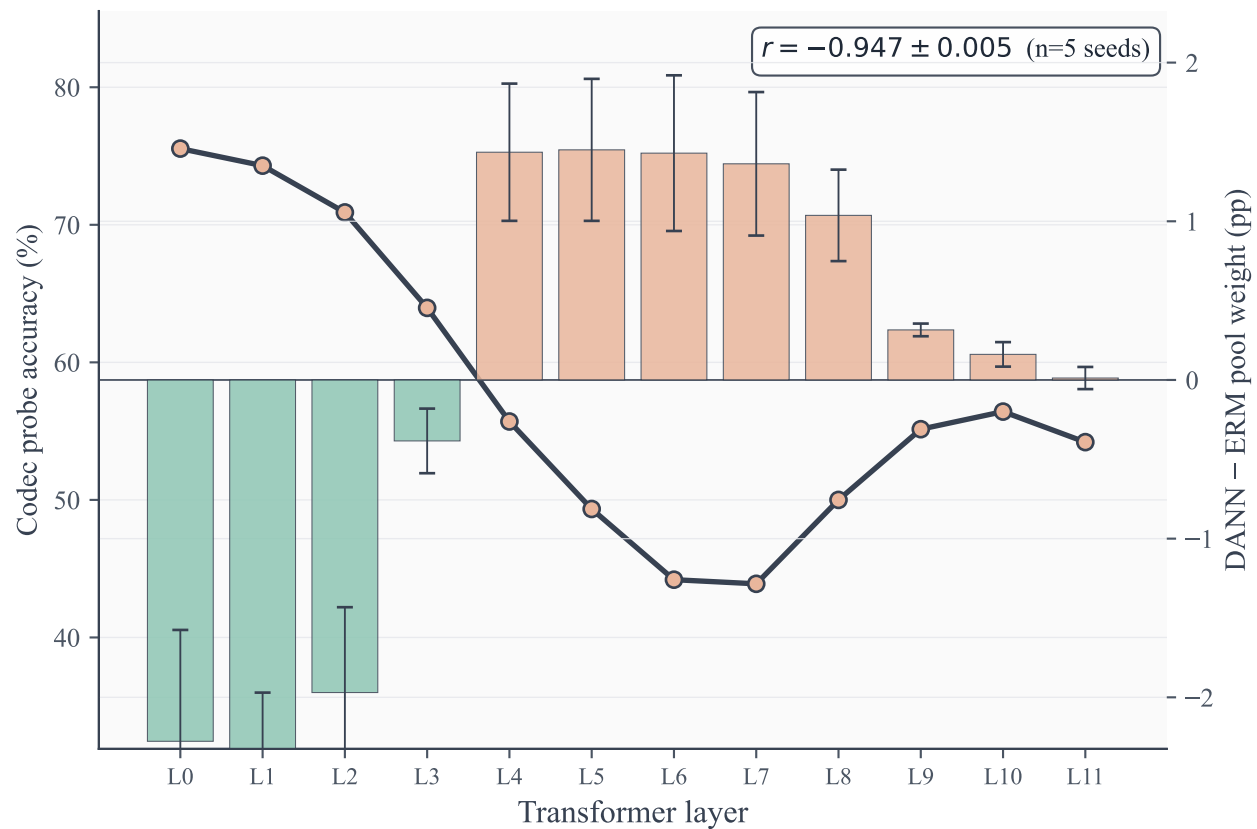
Wav2Vec 2.0
