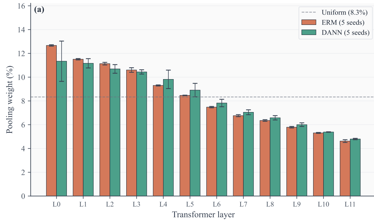
WavLM — weight shift
