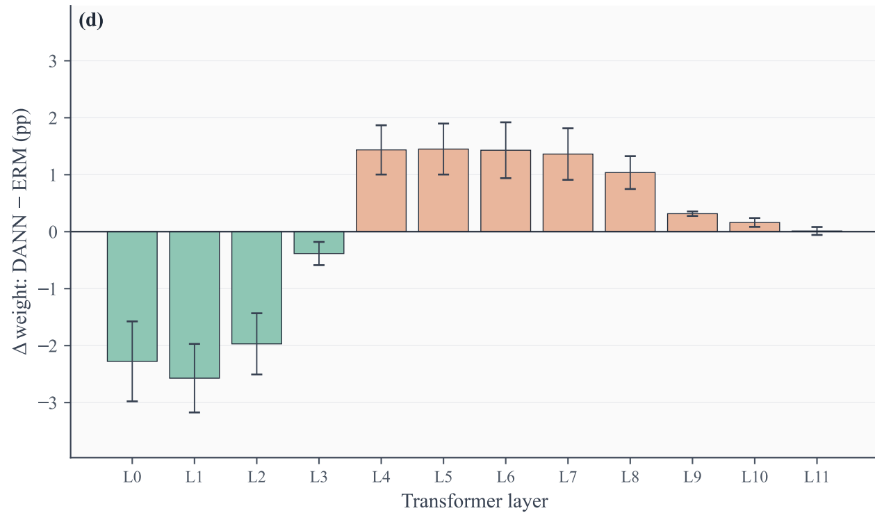
Wav2Vec 2.0 — weight shift
