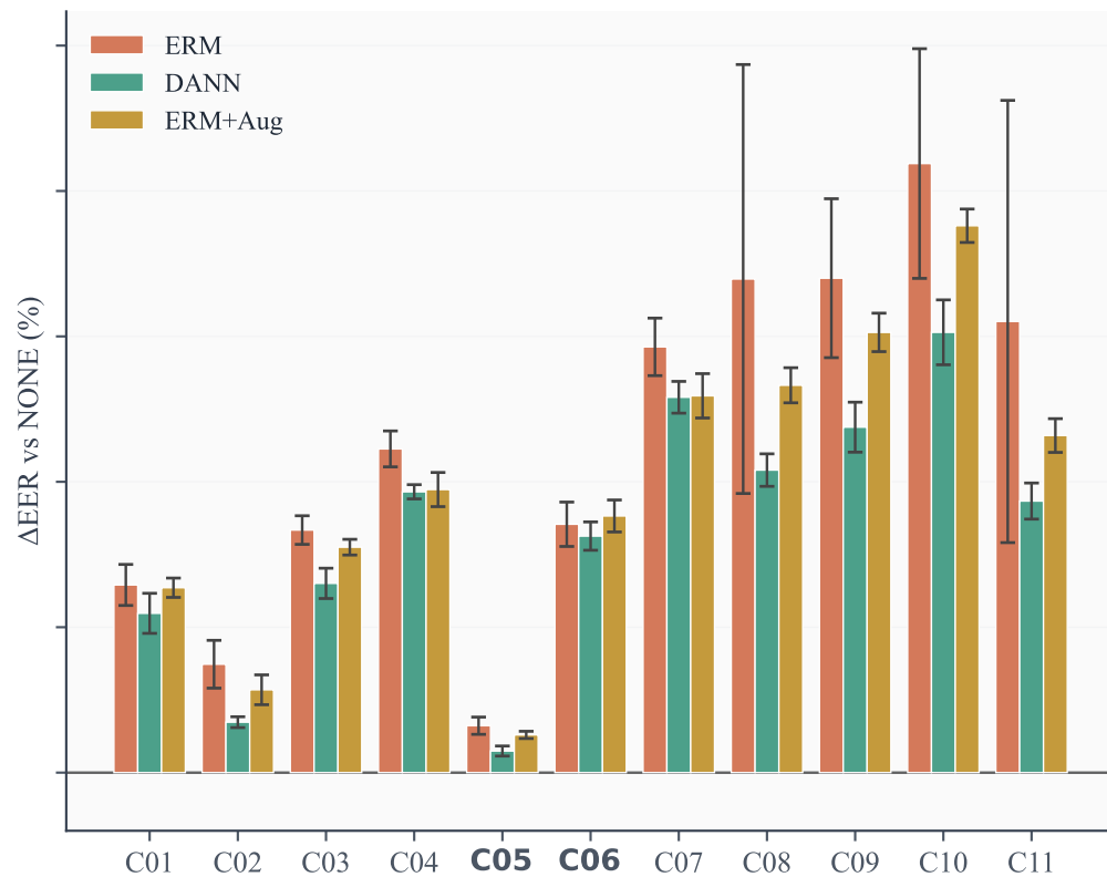
Wav2Vec 2.0
