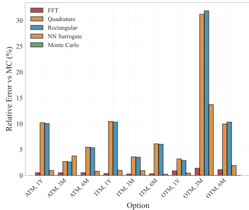
(d) Relative Error by Option Type
