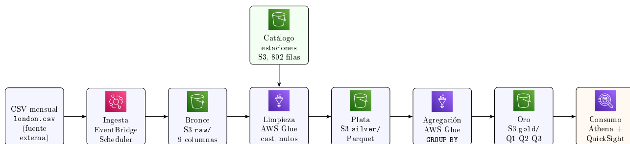
Figura 10: Pipeline ETL propuesto sobre AWS, capas medallón (bronce/plata/oro), con íconos oficiales de los servicios (Amazon S3, AWS Glue, Amazon EventBridge Scheduler, Amazon Athena) y entrada lateral del catálogo de estaciones en la etapa de limpieza.
