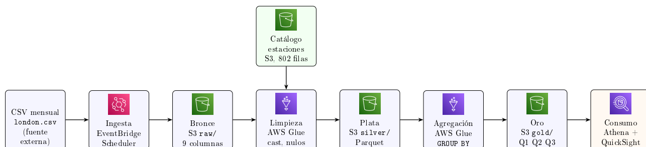
Figura 10: Pipeline ETL propuesto sobre AWS, capas medallón (bronce/plata/oro), con íconos oficiales de los servicios (Amazon S3, AWS Glue, Amazon EventBridge Scheduler, Amazon Athena) y entrada lateral del catálogo de estaciones en la etapa de limpieza.
