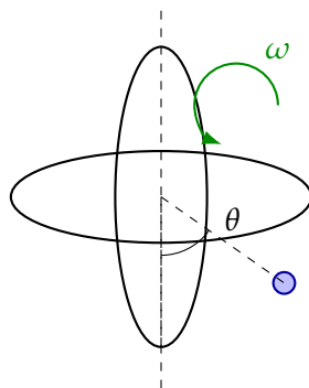
Figur 2.1: Perle (blå) på en cirkulær ring, der roterer med konstant vinkelhastighed \omega om den lodrette akse. Perlens eneste frihedsgrad er vinklen \theta målt fra ringens laveste punkt.
