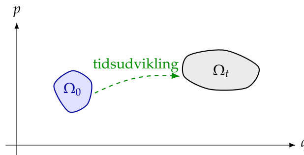
Figur 4.1: Liouvilles sætning: et område \Omega_0 i faserummet deformeres under tidsudviklingen til \Omega_t — formen ændres, men arealet (i to dimensioner) hhv. volumenet (i 2n dimensioner) er bevaret.
