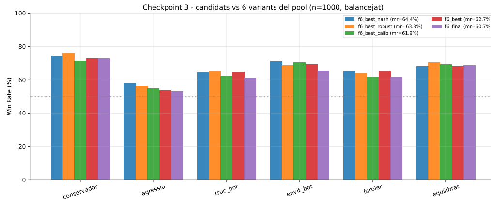
Figura A.8: Win-rate de cada candidat contra les sis variants del pool (1 000 partides balancejades). f6_best_nash (blau) assolix la metric_robust més alta (64,4%) i és el model seleccionat.
