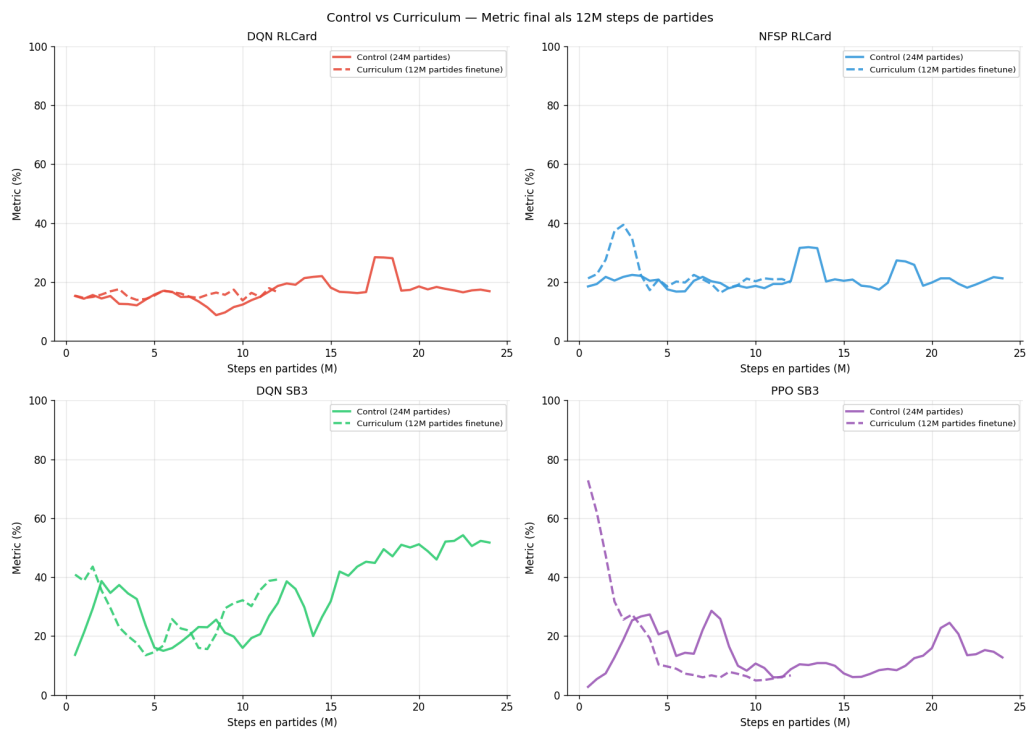
Figura A.4: Control vs currículum al final de l'etapa de partides (12M passos de finetune ). El currículum (línia discontinua) degrada els agents SB3 per sota del seu control, evidenciant l'oblit catastròfic.
