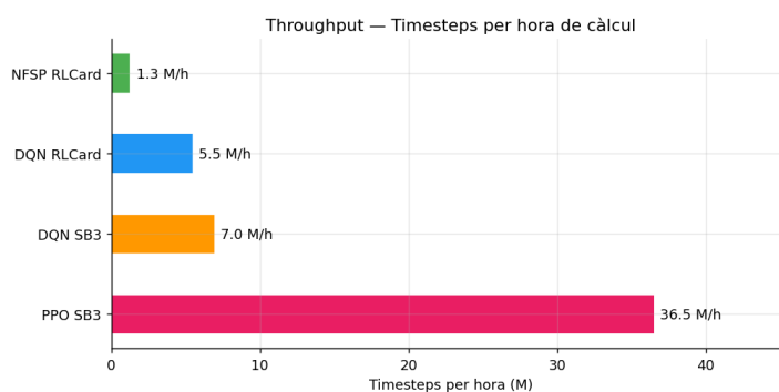
Figura A.1: Velocitat d'entrenament en milions de passos per hora de càlcul. PPO-SB3 és 28 vegades més ràpid que NFSP-RLCard gràcies al paral·lelisme de múltiples entorns.
