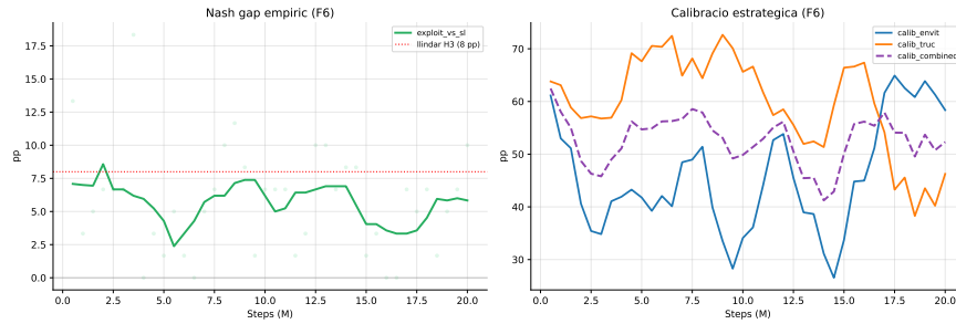
Figura 5.13: Panell esquerre: trajectòria del Nash gap empíric ( exploit_vs_sl ) amb llinar de 8 pp. Panell dret: evolució de la calibració estratègica ( calib_envit , calib_truc i calib_combined ).
