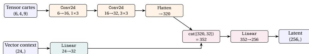
Figura 5.5: CosMultiInput : arquitectura de dues branques. La branca CNN processa el tensor de cartes (6, 4, 9); la branca lineal el vector de context (24,). Les sortides es concatenen i es projecten a un vector latent de 256 dimensions.
