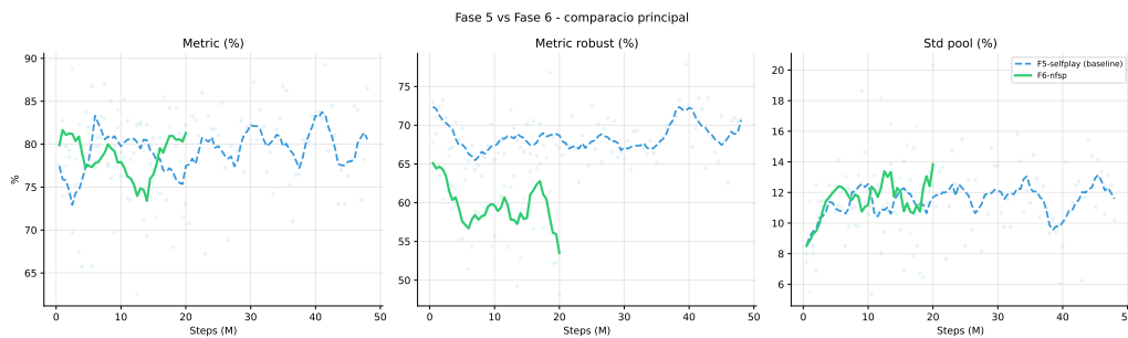
Figura 5.12: Corbes principals de F6-NFSP en tres panells: metric , metric_robust i std_pool , amb F5-selfplay com a referència discontinua. La inicialització amb els pesos de F5 accelera el pic inicial de metric , però la robustesa i la dispersió mostren estabilització més lenta fins a l'aturada anticipada als 20M passos.
