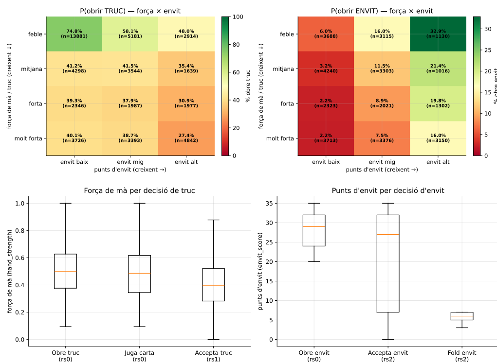
Figura 6.1: Política condicionada a la qualitat de la mà. A dalt, probabilitat d'obrir truc (esquerra) i d'obrir envit (dreta) segons la força de la mà (files) i els punts d'envit (columnes). A baix, distribució de la força de la mà per a les decisions de truc (esquerra) i dels punts d'envit per a les decisions d'envit (dreta). El truc és independent de la força (farol); l'envit hi està fortament lligat.
