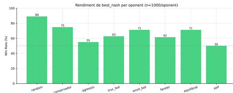
Figura A.11: Win-rate de best_nash contra cada oponent (1 000 partides per oponent). L'oponent agressiu és el més difícil (55%); contra si mateix el resultat és del 50%, consistent amb l'equilibri de Nash.
