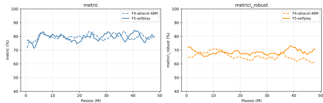
Figura 5.10: Evolució de la metric (esquerra) i la metric_robust (dreta) al llarg de 48M passos. Línia discontinua: F4-ablació-48M (sense self-play); línia sòlida: F5-selfplay. La metric és pràcticament idèntica (H1), però la metric_robust de F5 creix de forma sostinguda i supera àmpliament la de F4 (H2).
