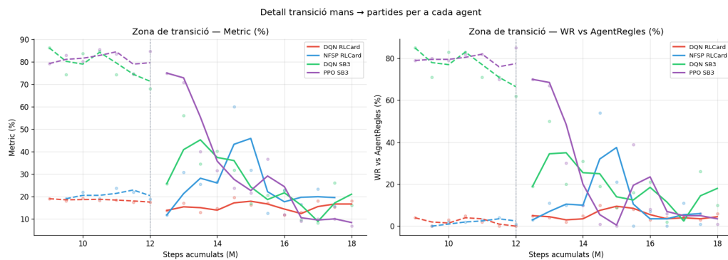
Figura A.5: Detall de la zona de transició mans → partides. La línia puntejada vertical marca el canvi de protocol (12M passos). PPO-SB3 mostra la caiguda més dràstica: de 80% a menys del 10% en pocs checkpoints.
