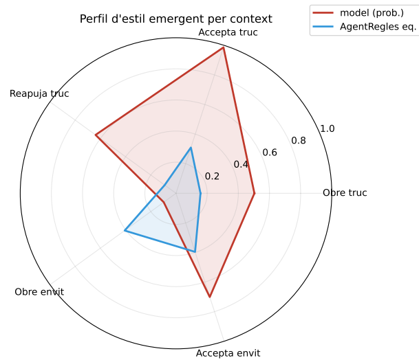
Figura A.13: Perfil d'estil emergent del model desplegat (vermell) comparat amb l'agent basat en regles equilibrat (blau) en cinc dimensions de context. El model mostra una agressió al truc superior i una propensió a l'envit inferior a la de l'agent de regles.
