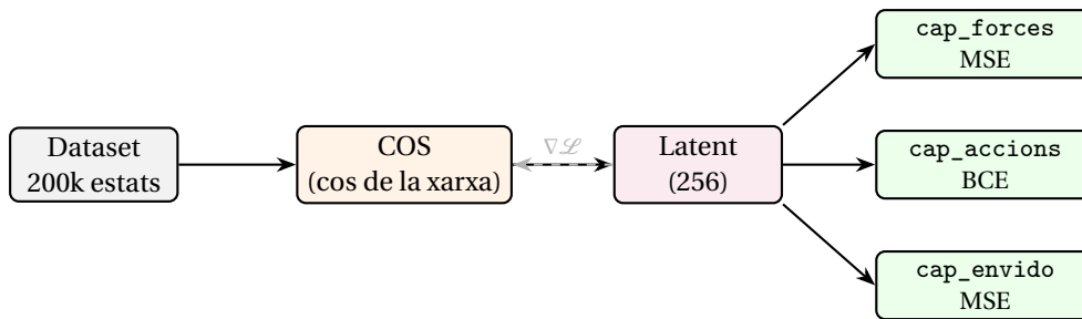
Figura 5.6: Esquema del preentrenament supervisat: els tres caps propaguen gradient al cos i l'obliguen a aprendre representacions sensibles a l'estructura del joc. Un cop acabat, els caps es descarten i es conserven només els pesos del cos.
