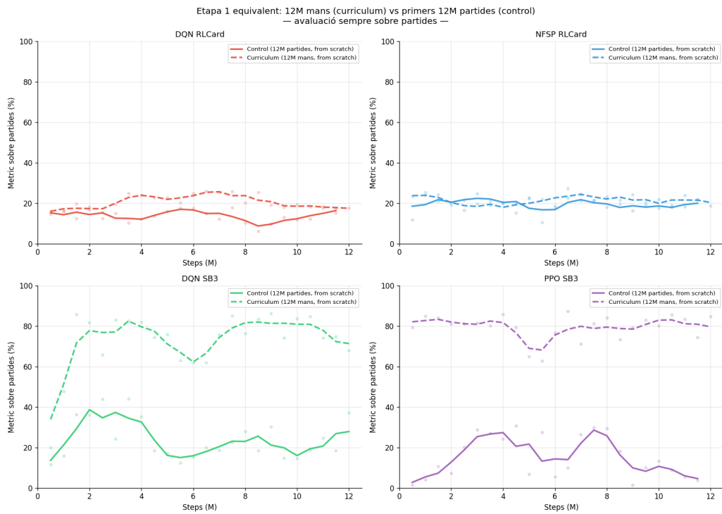
Figura A.3: Comparació de l'etapa 1 equivalent: 12M passos sobre mans (currículum) contra els primers 12M passos directament sobre partides (control). En els agents SB3, les mans eleven la mètrica molt per sobre del control; en els de RLCARD la diferència és mínima.
