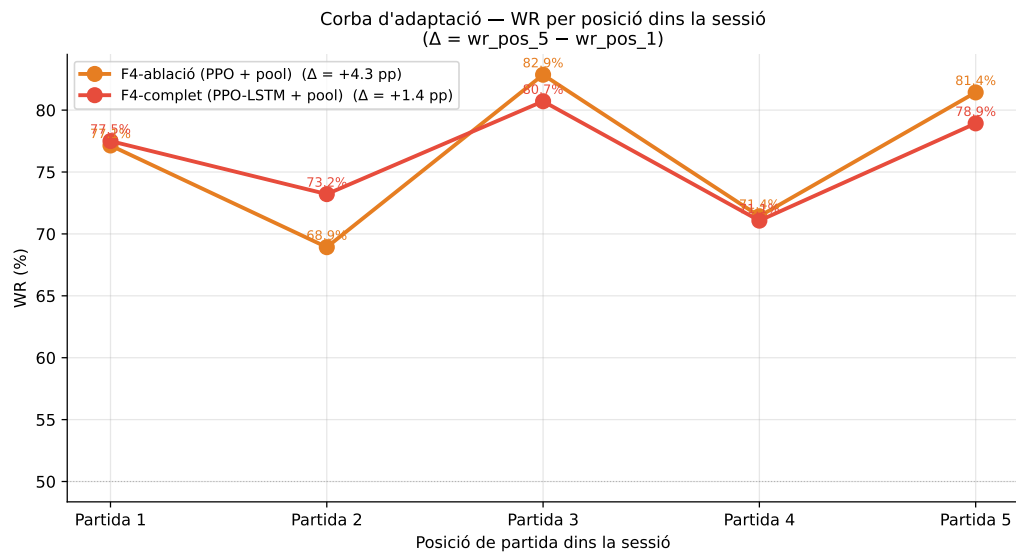
Figura 5.8: Win-rate per posició dins la sessió (mà 1 a mà 5) per als dos entrenaments de la Fase 4 (mitjana de les cinc darreres avaluacions). El \Delta indica la diferència entre la mà 5 i la mà 1. La línia puntejada marca el 50%.
