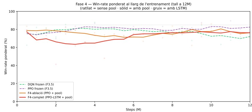
Figura 5.7: Evolució del win-rate ponderat (metric) al llarg de l'entrenament per als quatre entrenaments de la Fase 4, tallats a 12M passos. Línies discontinúes: línies base de la Fase 3.5 (sense pool); línies sòlides: entrenaments amb pool; gruix addicional: model amb LSTM. La línia puntejada gris marca el 85%.
