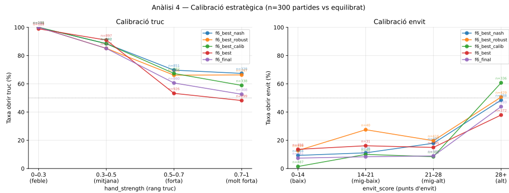
Figura A.10: Taxa d'obrir truc per franja de força de mà (esquerra) i taxa d'obrir envit per puntuació d'envit (dreta) dels cinc candidats (300 partides vs agent equilibrat). Tots mostren el patró de farol al truc (decreixent amb la força) i una política d'envit creixent amb la puntuació; les diferències entre candidats són petites, cosa que confirma que la selecció es basa en el Nash gap i no en el comportament qualitatiu.
