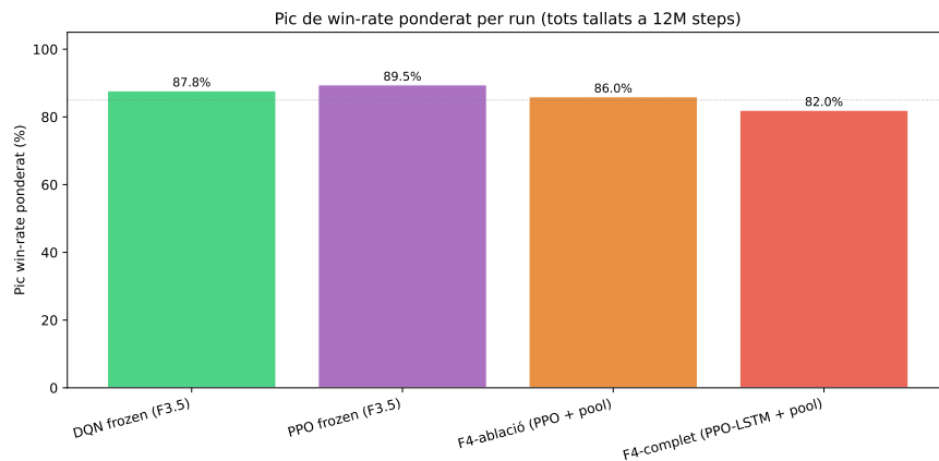
Figura A.7: Pic de win-rate ponderat per als quatre entrenaments de la Fase 4, tots tallats a 12M passos. PPO frozen (F3.5) assoleix el màxim (89,5%), seguit de DQN frozen (87,8%). L'afegit de LSTM (F4-complet) no millora el pic en aquest pressupost.
