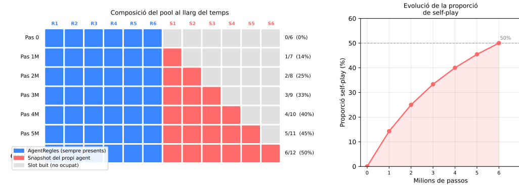
Figura 5.9: Composició del pool mixt al llarg del temps. Esquerra: cada fila és un instant clau; les caselles blaves (R1–R6) són les sis variants de l’agent basat en regles, sempre presents; les caselles vermelles (S1–S6) són les versions de pesos anteriors del propi agent, afegides una a una cada milió de passos. Dreta: evolució de la proporció de self-play, que passa de 0% al pas 0 fins al 50% quan el pool és ple (pas 6M en endavant).
