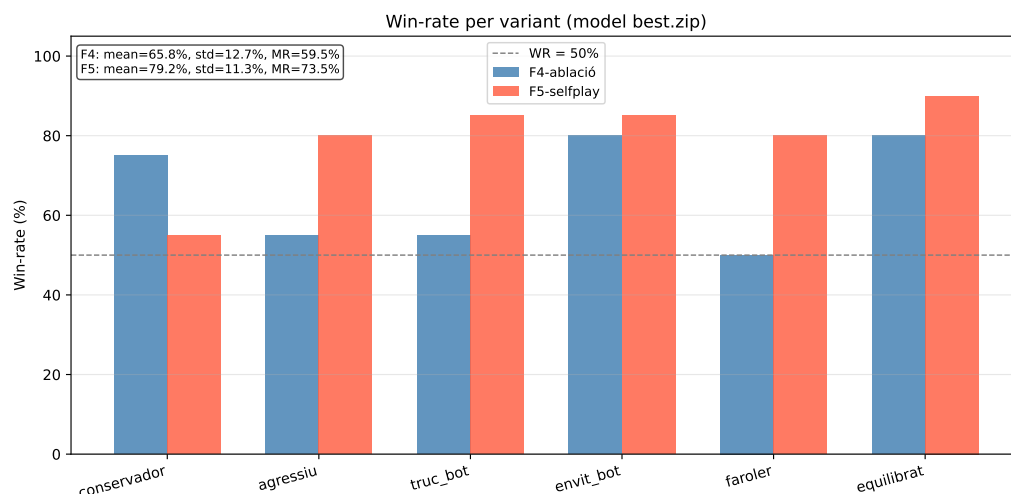
Figura 5.11: Win-rate per variant d'oponent (models seleccionats). F4 (blau) mostra una distribució irregular: alt contra l'estil conservador i equilibrat, baix contra l'agressiu i el faroler. F5 (vermell) reequilibra la distribució: puja tots els valors baixos al 80–85% al preu d'abaixar l'estil conservador (la variació inversa és el senyal que la política ja no s'especialitza).
