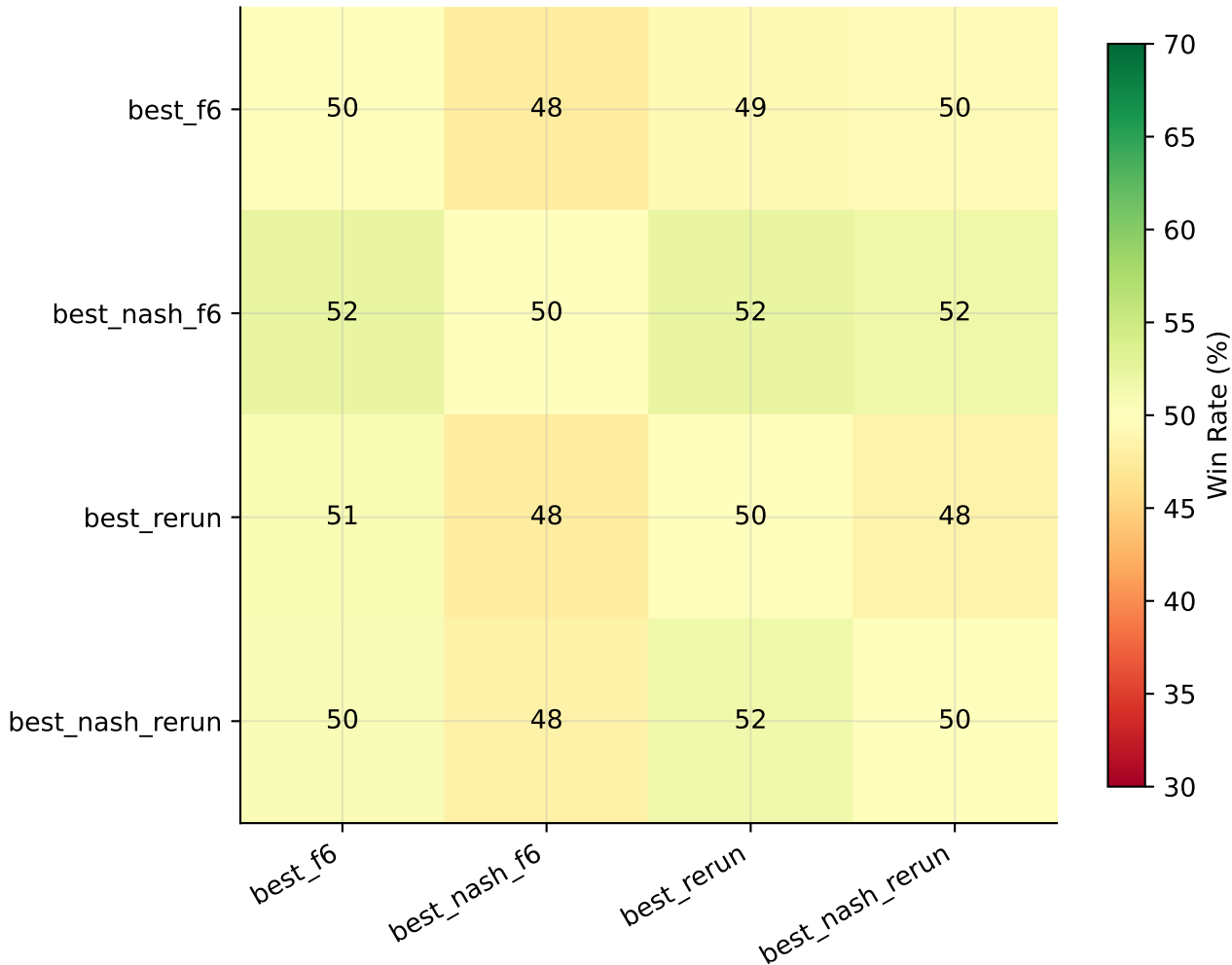
Round-robin: WR fila vs columna (%) (n=1000)
