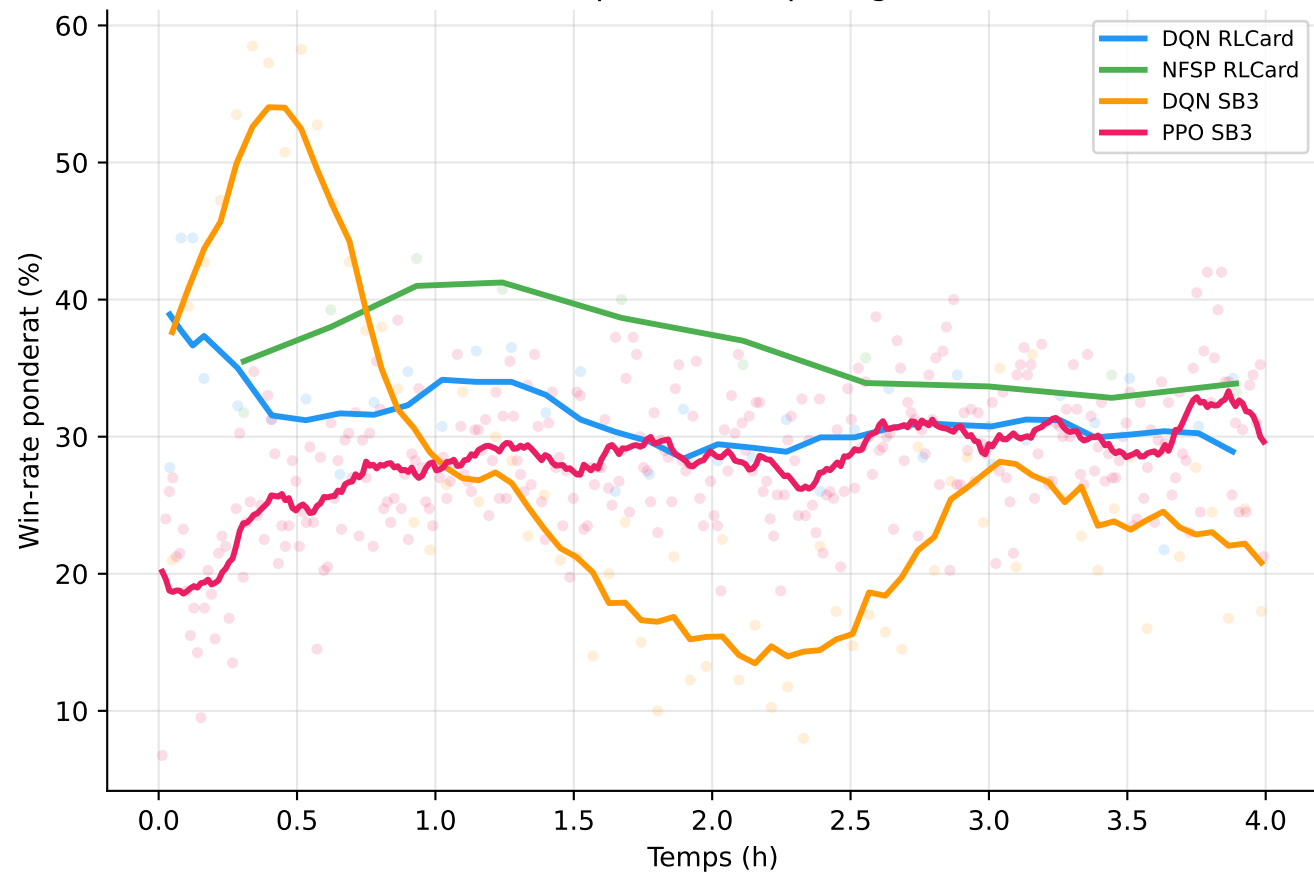
Per temps real (4 h per agent)
