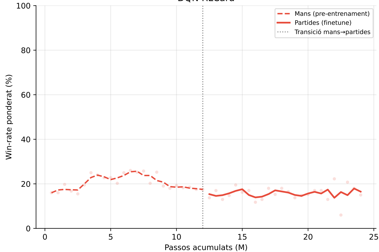
DQN RLCard
