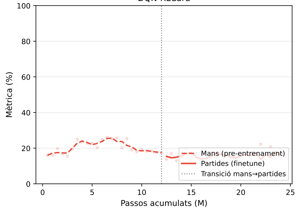
DQN-RLCard
