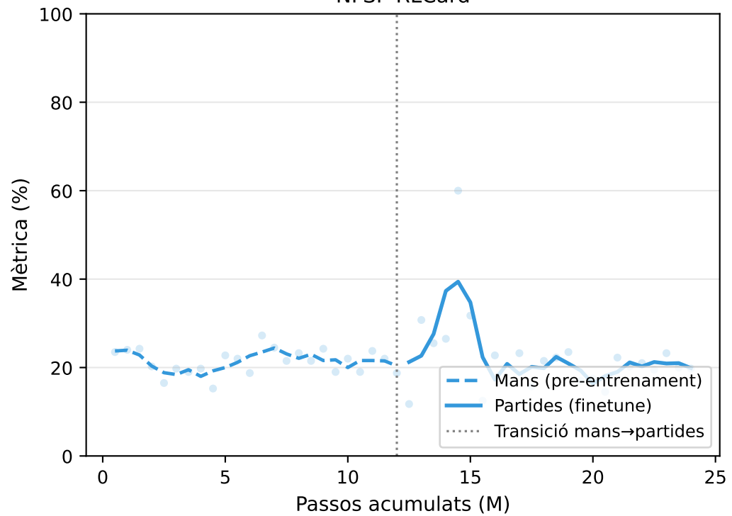
NFSP-RLCard
