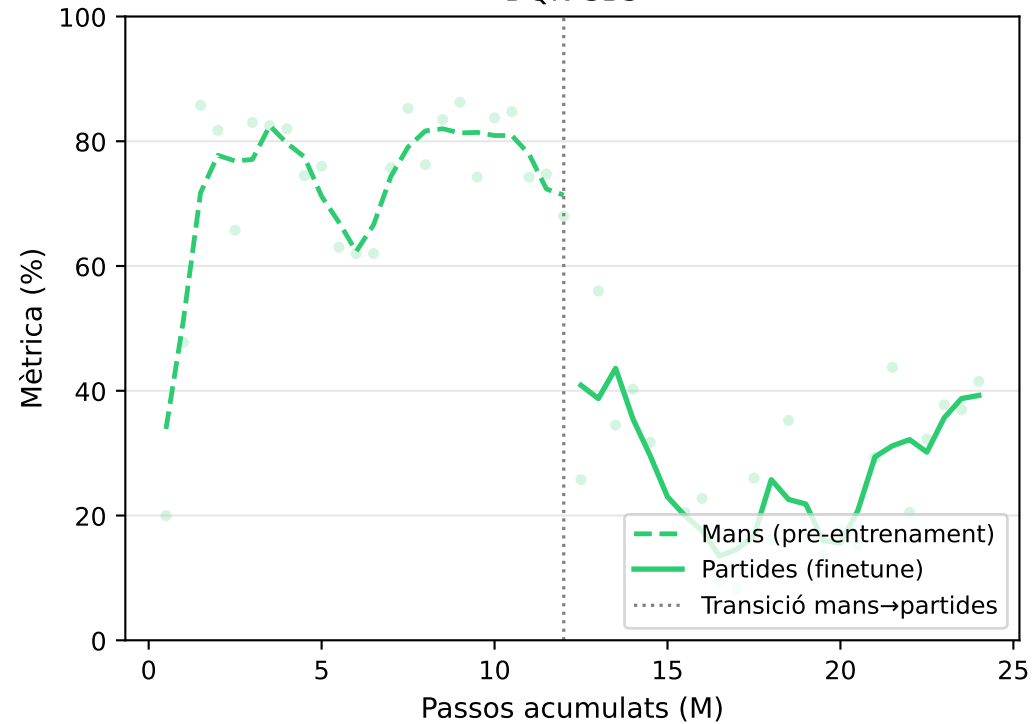
DQN-SB3
