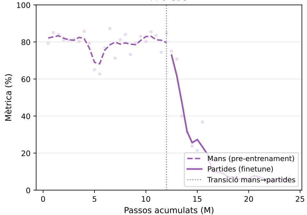
PPO-SB3
