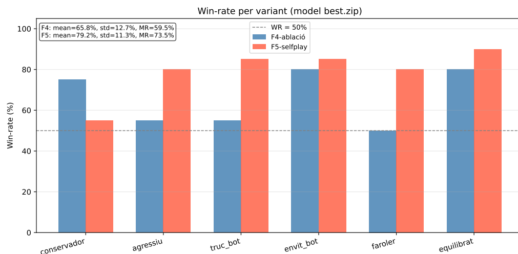
Figura 5.13: Win-rate per variant d'oponent (models best . zip). F4 (blau) mostra una distribució irregular: alt contra l'estil conservador i equilibrat, baix contra l'agressiu i el faroler. F5 (vermell) reequilibra la distribució: puja tots els valors baixos al 80–85% al preu d'abaixar l'estil conservador (la variació inversa és el senyal que la política ja no s'especialitza).
