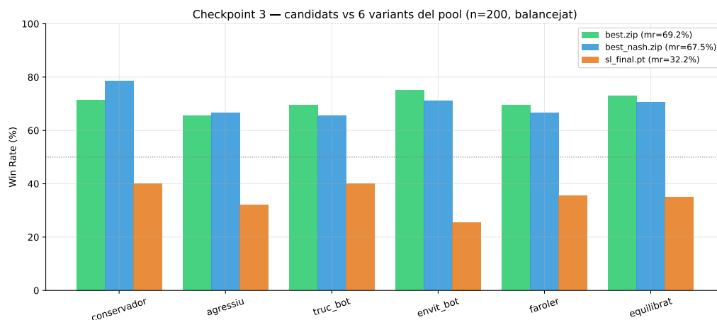
Figura 5.16: Win-rate dels tres candidats contra les 6 variants del pool (200 partides balancejades per variant). best.zip i best_nash.zip rendeixen gairebé igual; sl_final.pt (política mitjana SL) queda clarament per sota del 50 % a totes les variants.
