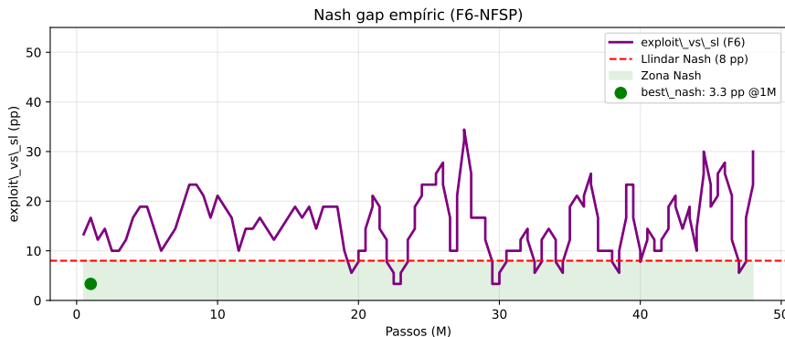
Figura 5.15: Nash gap empíric ( exploit_vs_sl ) al llarg de l'entrenament de F6. La línia discontinua vermella marca el llindar de 8 pp (criteri de H3); la zona verda mostra la zona Nash. El punt destacat correspon al checkpoint best_nash (3,3 pp @1M passos), l'únic moment on el sistema toca l'equilibri de forma clara.
