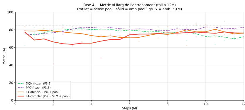
Figura 5.8: Evolució de la metric al llarg de l'entrenament per als quatre runs de la Fase 4, tallats a 12M passos. Línies discontinuïques: línies base de la Fase 3.5 (sense pool); línies sòlides: runs amb pool; gruix addicional: model amb LSTM. La línia puntejada gris marca el 85%.
