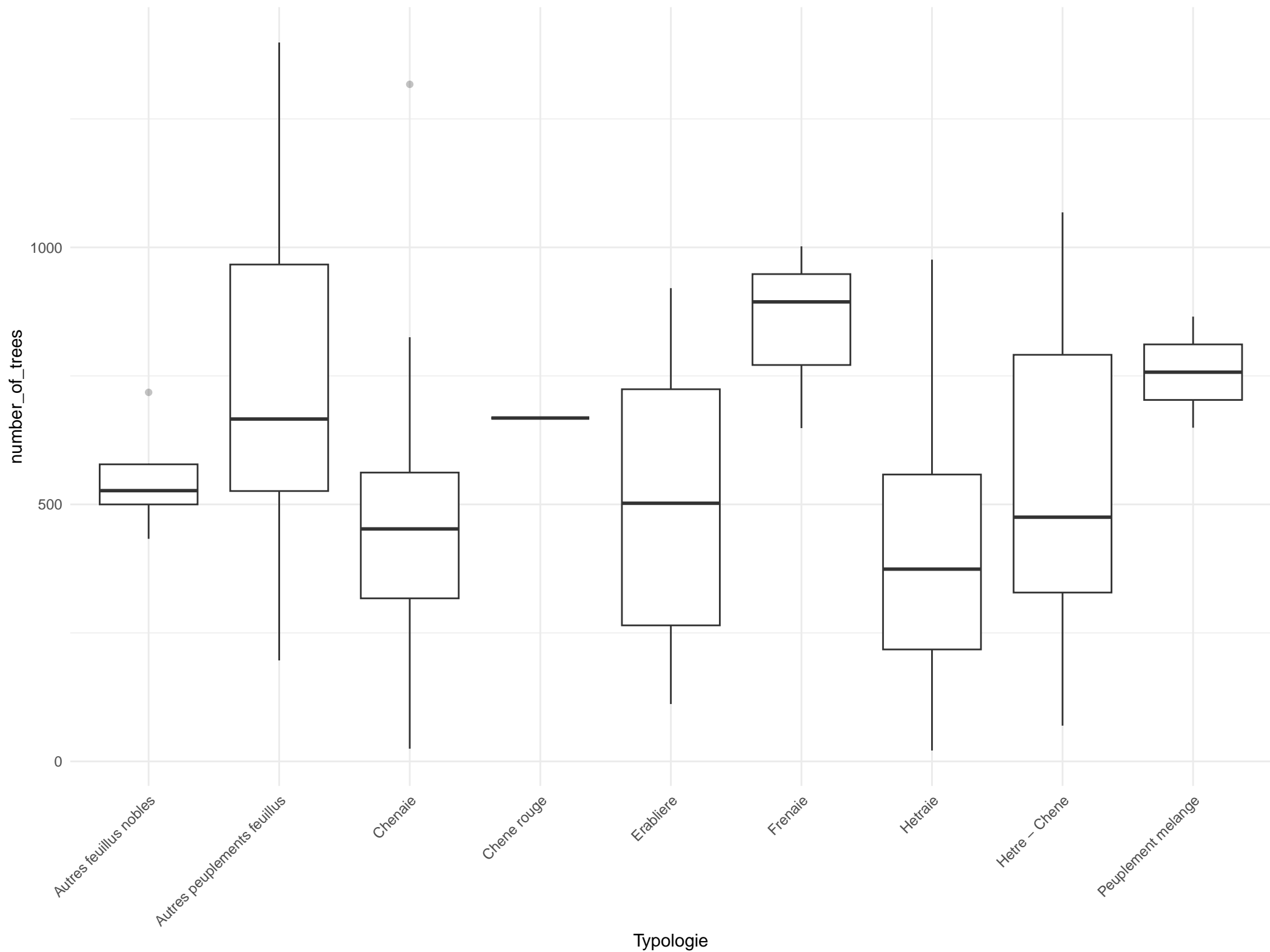
Boxplot de number_of_trees par typologie
