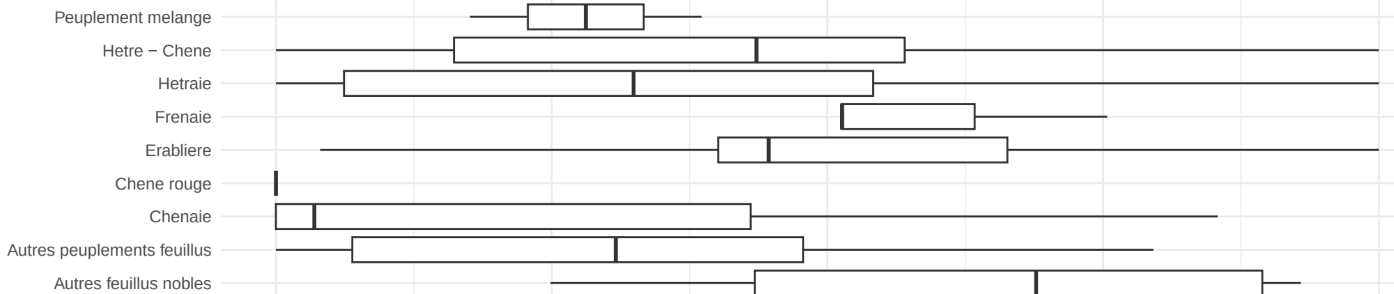
Gros bois couché (FAS)
