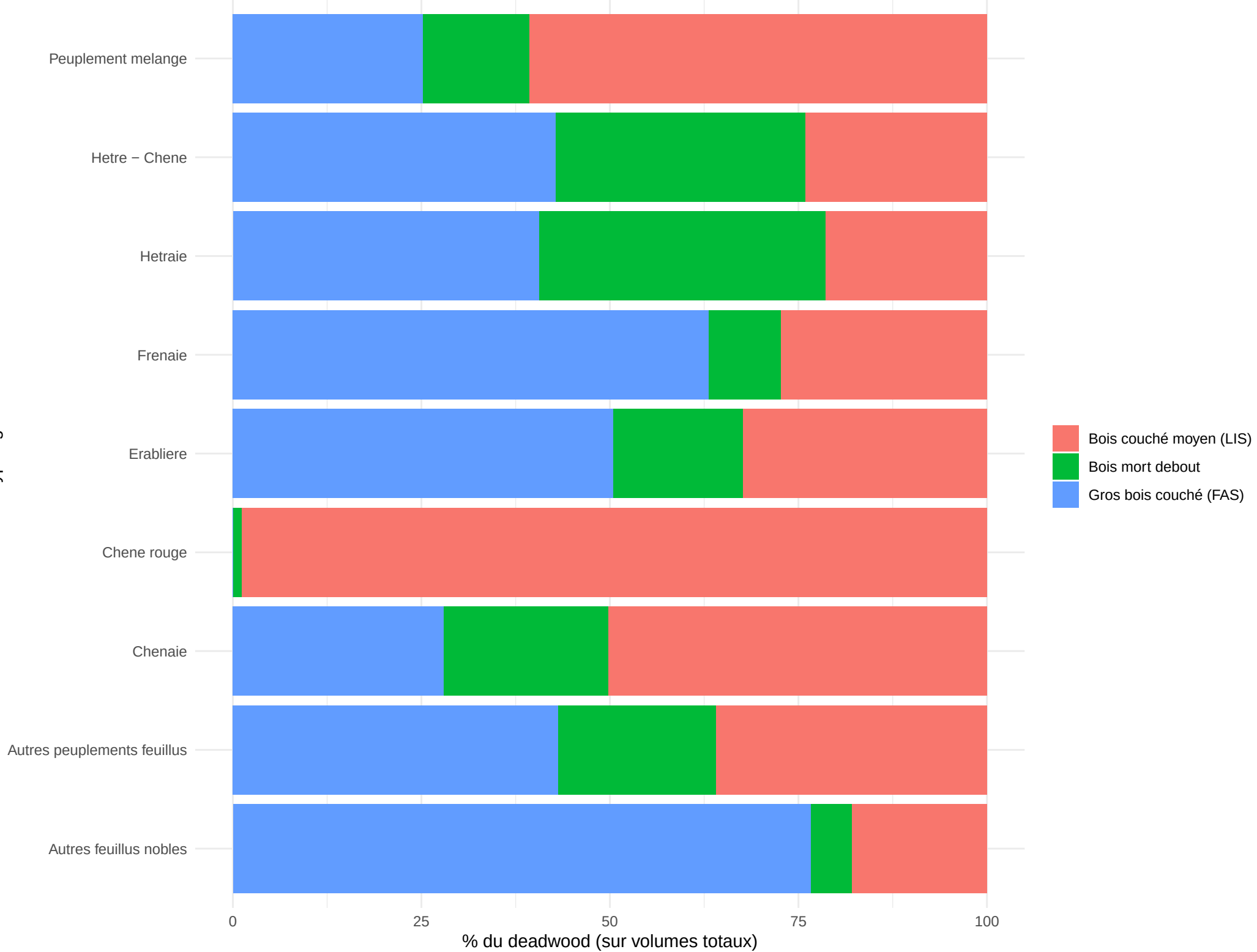
Deadwood par typologie : répartition (%)
