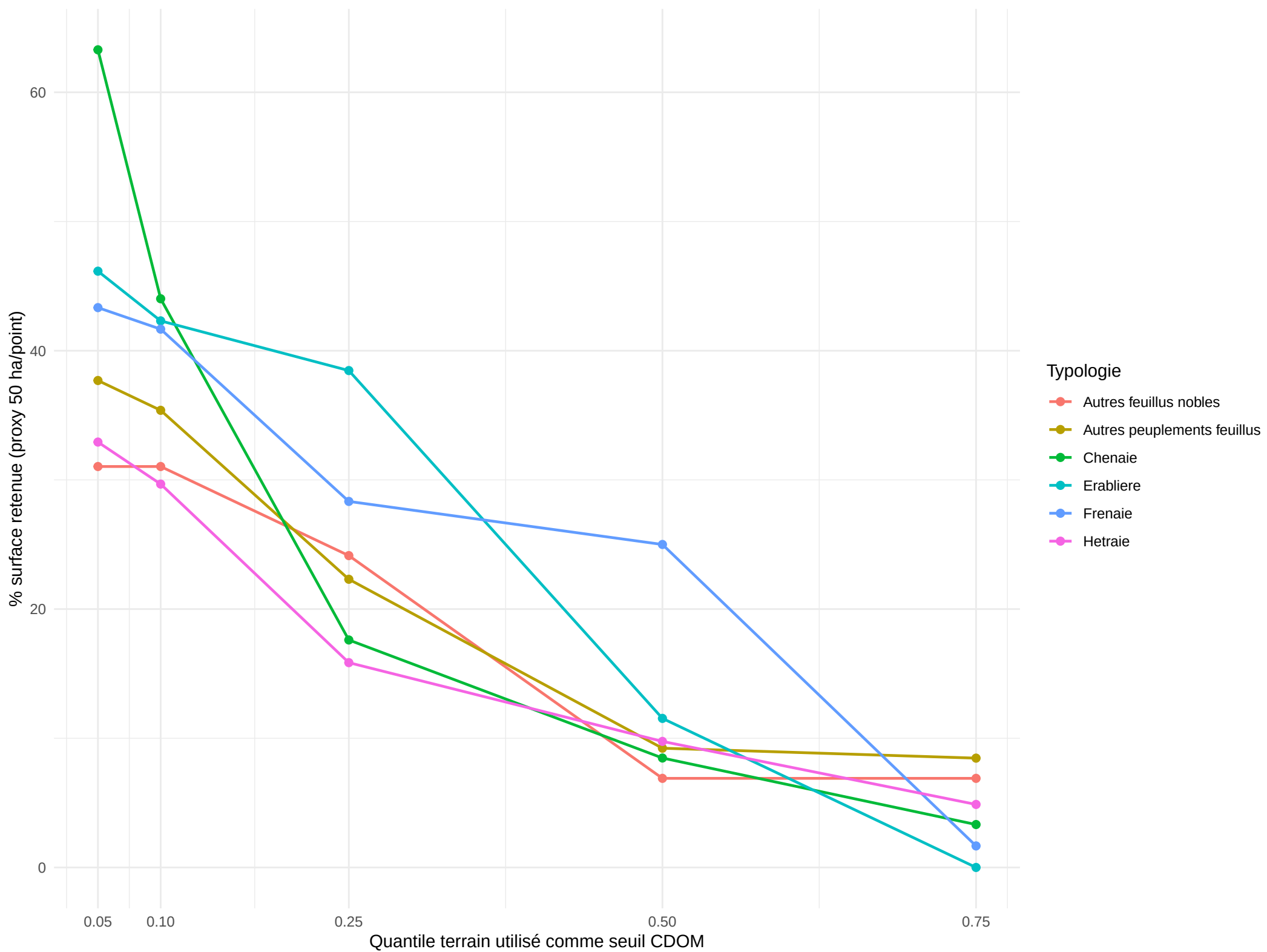
Sensibilité aux seuils CDOM — avant masque FA
