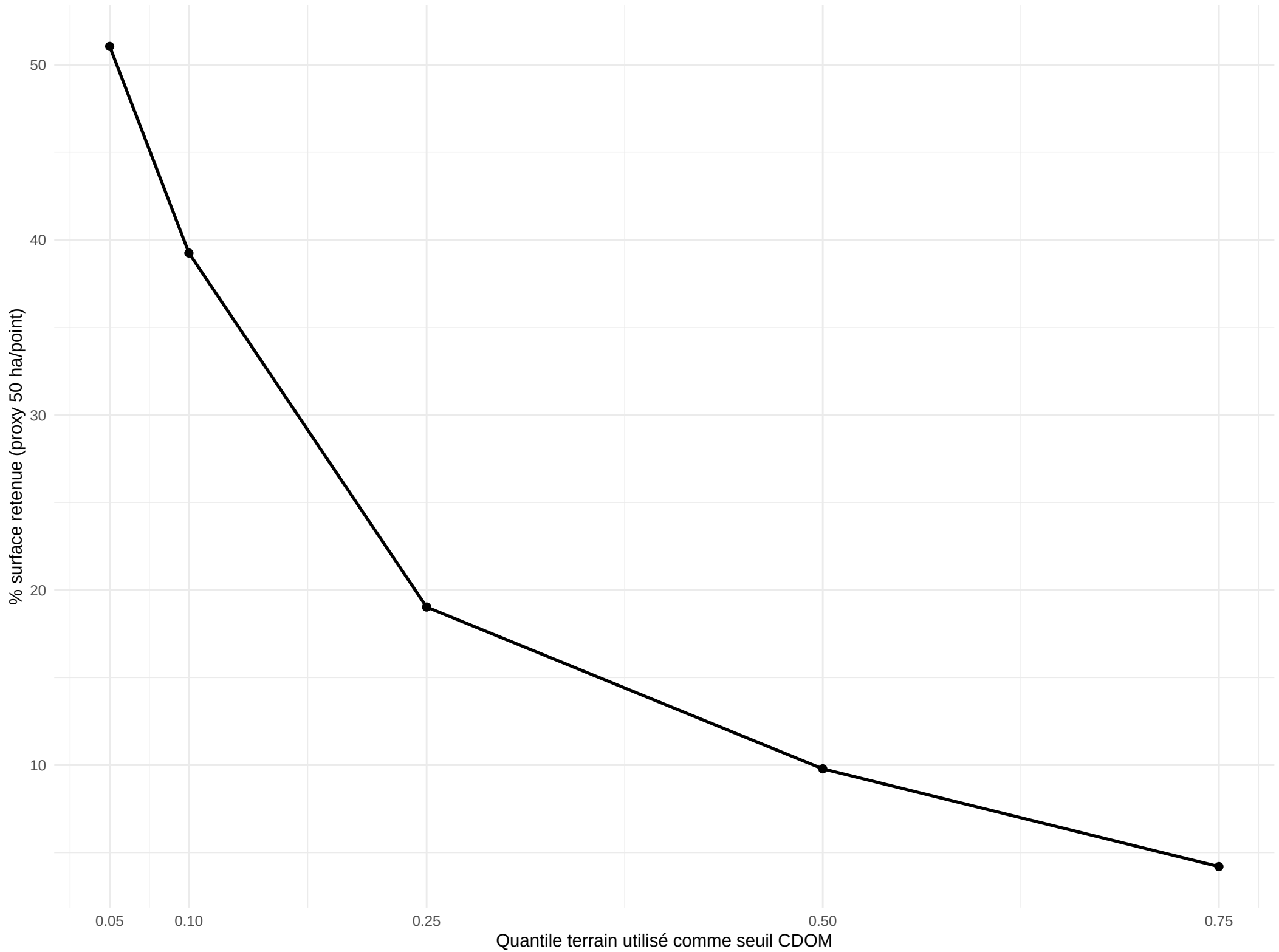
Sensibilité globale — avant masque FA
