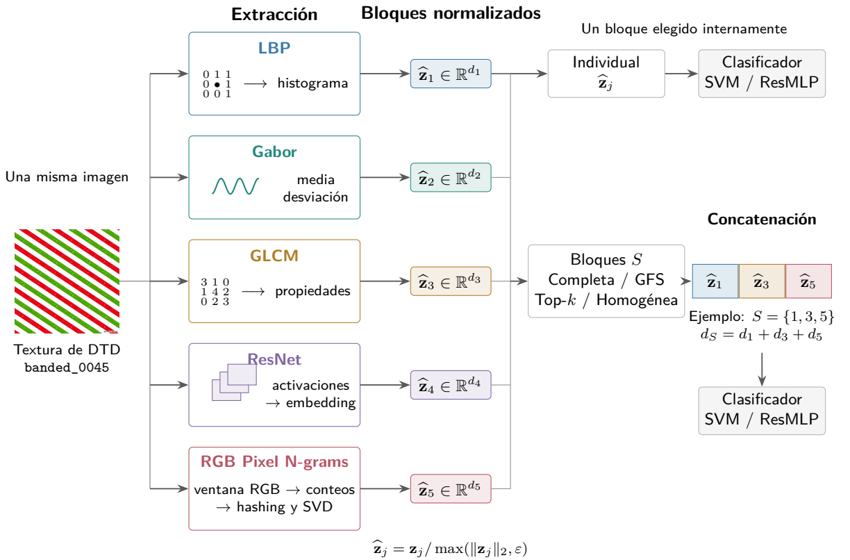
Figura 1: Extracción y concatenación de descriptores. La misma imagen de DTD se representa mediante cinco ejemplos: patrones locales (LBP), respuestas de filtros (Gabor), coocurrencias (GLCM), una red convolucional (ResNet) y secuencias RGB (N-gramas). Las transformaciones internas se muestran esquemáticamente; no representan mapas de importancia por píxel. Cada rama produce un bloque normalizado que puede utilizarse individualmente o concatenarse con otros. El ejemplo de tres bloques ilustra la unión de coordenadas; cada política determina el subconjunto admisible.
