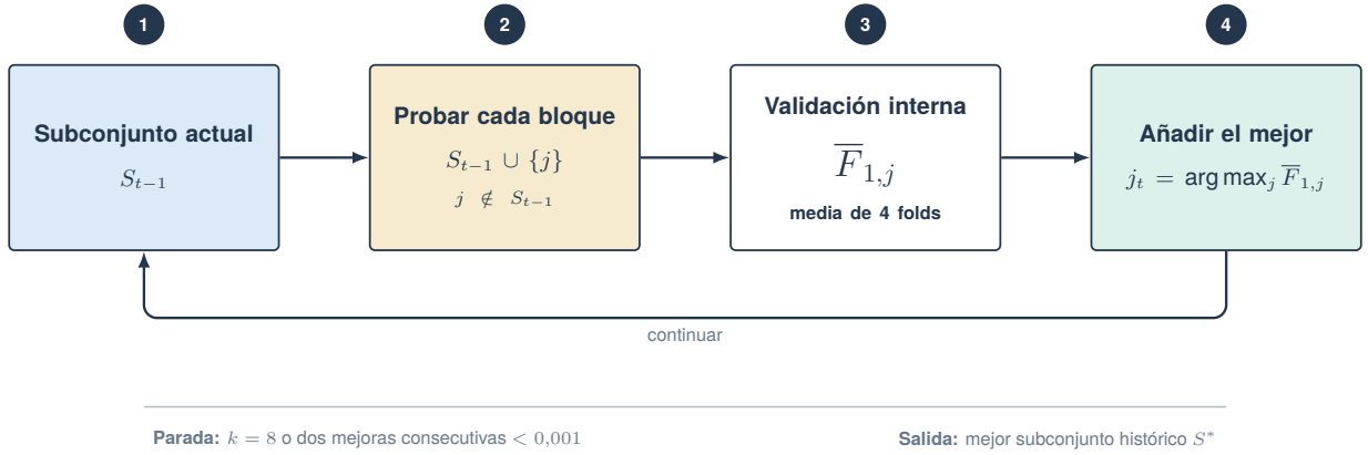
Figura 2: Mecanismo de Greedy Forward Selection sobre bloques completos. En cada paso se elige el bloque que maximiza el macro-F1 medio de la validación interna; el test externo se utiliza únicamente tras cerrar el subconjunto.
