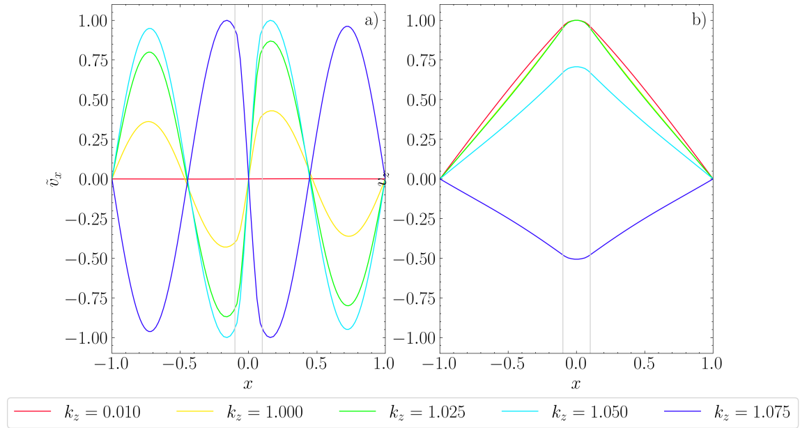
Figura 9: Evolució de les autofuncions del primer mode ràpid aprop de l'anticreuant evitat.
