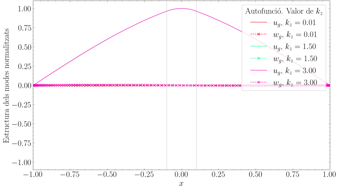
Figura 10: Evolució de les autofuncions del mode fHL.
