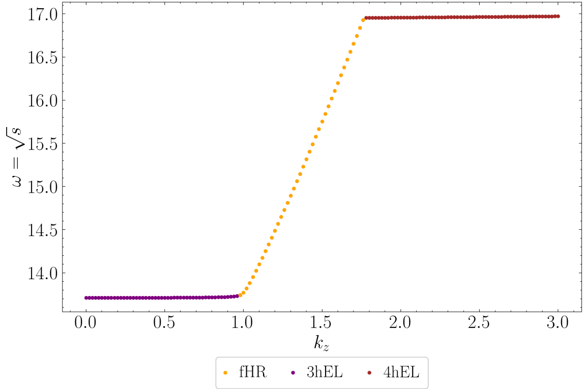
Figura 6: Evolució d'un mode normal individual ( n = 5 ).
