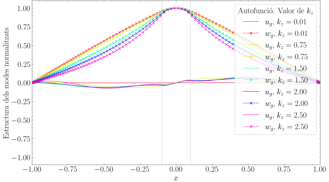
Figura 11: Evolució de les autofuncions del mode fHR.
