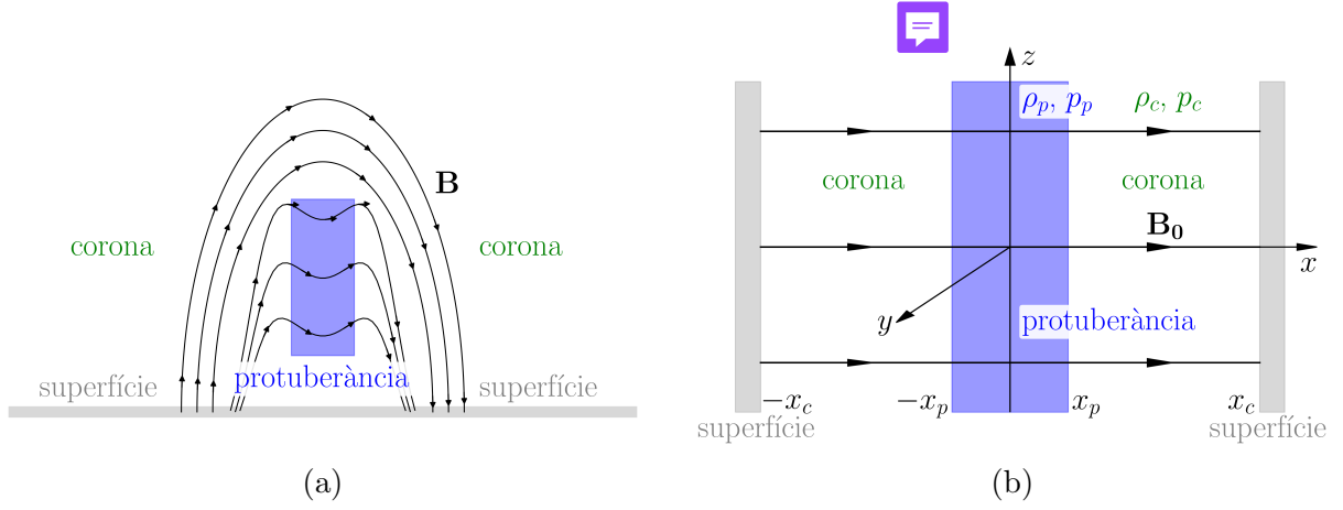
Figura 1: (a) Representació esquemàtica d'una protuberància solar en la corona. (b) Diagrama del sistema en equilibri tèrmic, com a làmina plana paral·lela a la superfície amb dimensions de 2x_p de gruix en direcció \hat{x} , d'alçada infinita en direcció \hat{z} i infinita en direcció \hat{y} . El camp magnètic quiescent, \mathbf{B}_0 , és horitzontal, en direcció \hat{x} . L'elecció dels eixos s'ha fet amb l'objectiu que el vector d'ona sigui normal al camp magnètic estàtic i paral·lel a la direcció de la protuberància.
