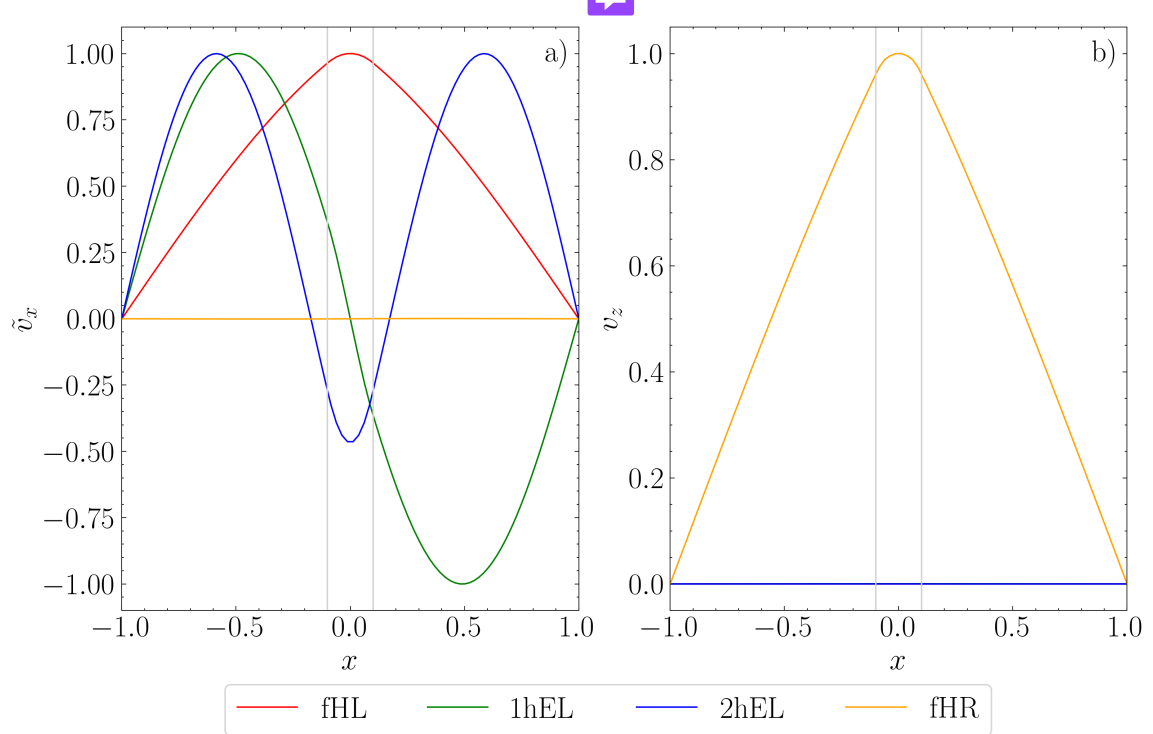
Figura 8: Estructura de les autofuncions associades als primers 4 modes per k_z = 0.01 .
