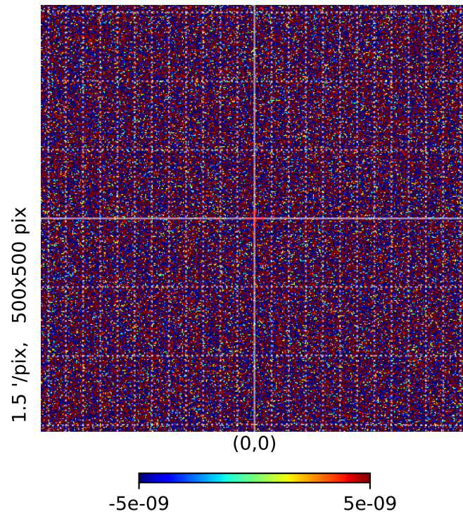
\mu y P-CILC reconstruction
