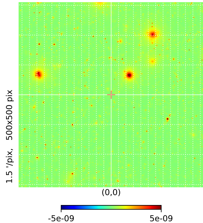
\mu y input signal
