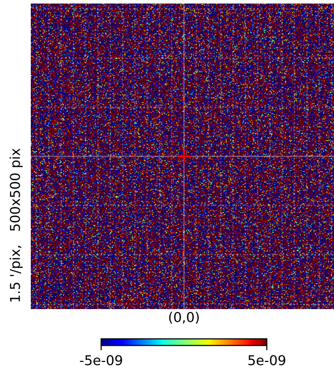
\mu y residual (input - P-CILC)
