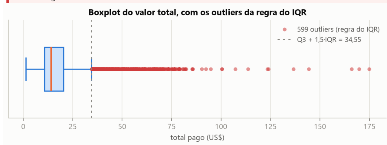
Figura 2 — Boxplot do valor total com as cercas de Tukey e os outliers destacados.
